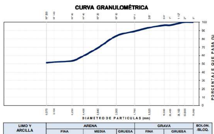
Figura 24 Curva granulométrica de la muestra 1.
