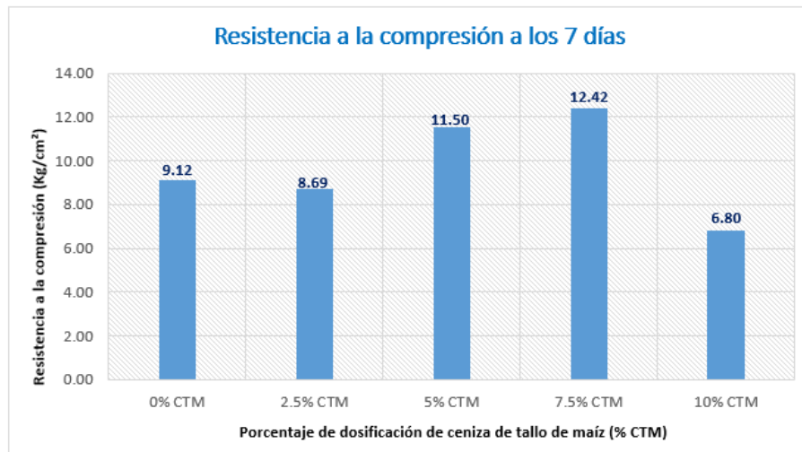
Figura 53 Resultados promedio del ensayo de la resistencia a la compresión (Kg/cm 2 ) a los 7 días.
