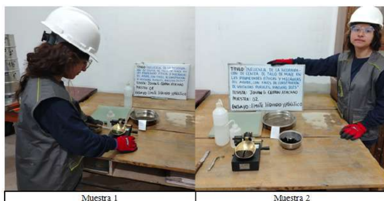
Figura 20 Muestra 1 y 2 para la determinación de límite líquido.
