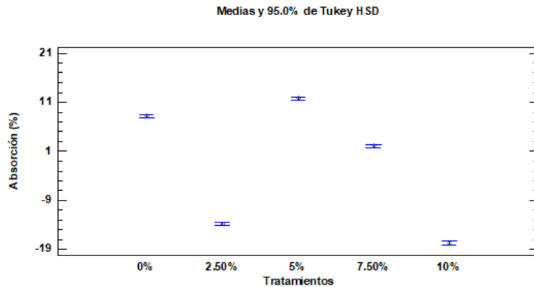
Figura 59 Gráfico de medias para Absorción (%) por tratamientos. Fuente: STATGRAPHICS - Elaboración propia
