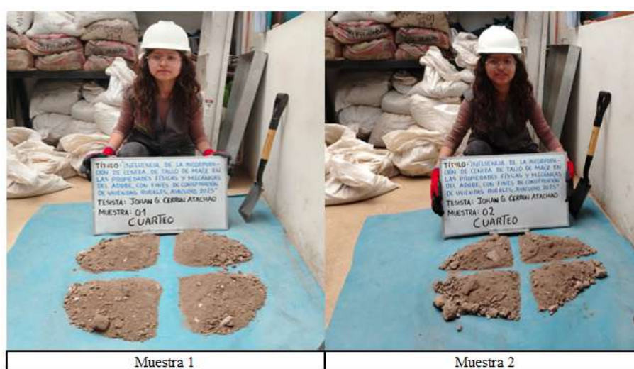
Figura 16 Cuarteo de la muestra 1 y 2 de suelo.
