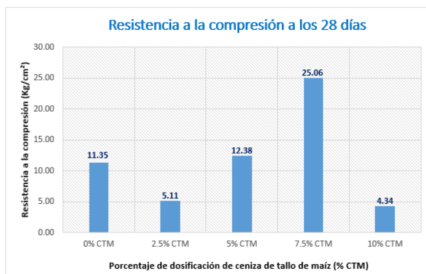
Figura 55 Resultados promedio del ensayo de la resistencia a la compresión (Kg/cm 2 ) a los 28 días.
