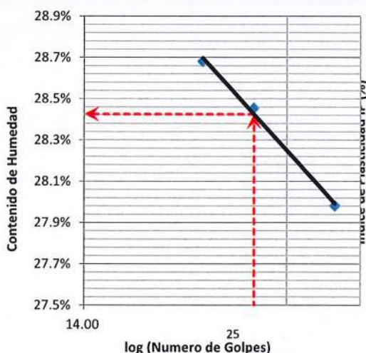
CURVA DE FLUIDEZ
