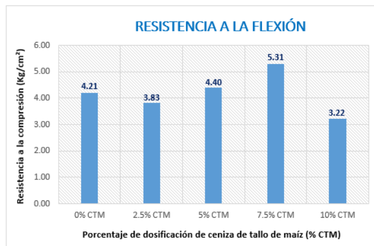
Figura 58 Resultados promedio del ensayo de la resistencia a la flexión (Kg/cm 2 ).
