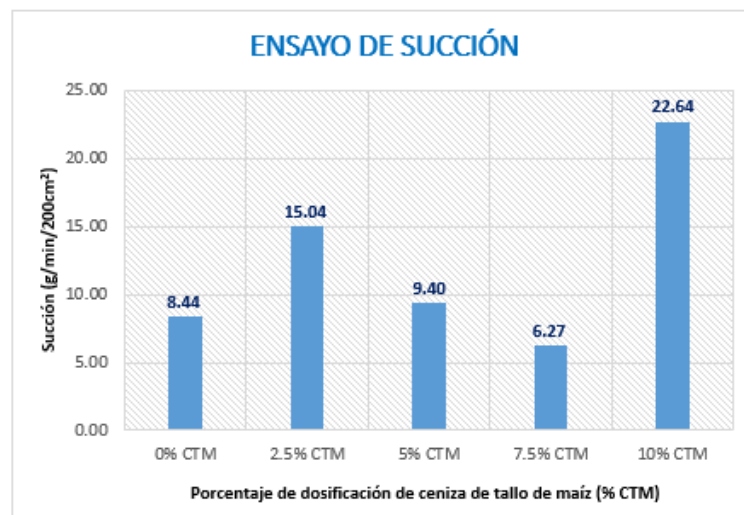
Figura 51 Resultados promedio del ensayo de succión ( \text{g/min/200cm}^2 ).
