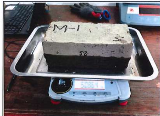
Figura 02: Peso de muestra saturada M-1 con 2.5% de ceniza de tallo de maíz
