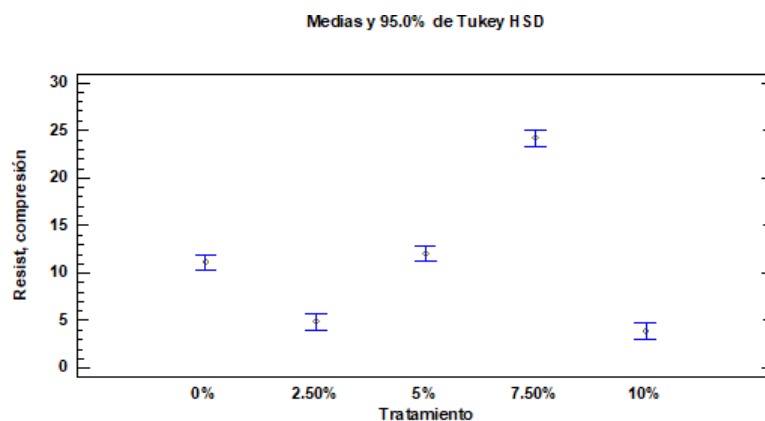
Figura 62 Gráfico de medias para Resistencia a la compresión a los 28 días adobe 10x10x10cm.
