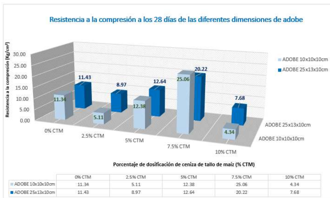
Figura 57 Comparación de los resultados promedio del ensayo de la resistencia a la compresión de las unidades de 25x13x10cm y 10x10x10cm a los 28 días.
