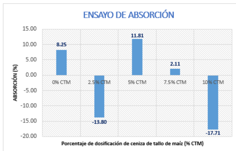
Figura 50 Resultados promedio del ensayo de absorción (%).
