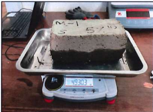
Figura 03: Peso de muestra saturada M-1 con 5% de ceniza de tallo de maíz
