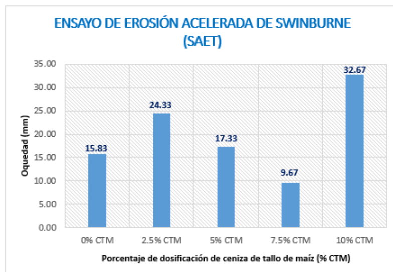
Figura 52 Resultados promedio del ensayo a la resistencia a la erosión acelerada (mm).
