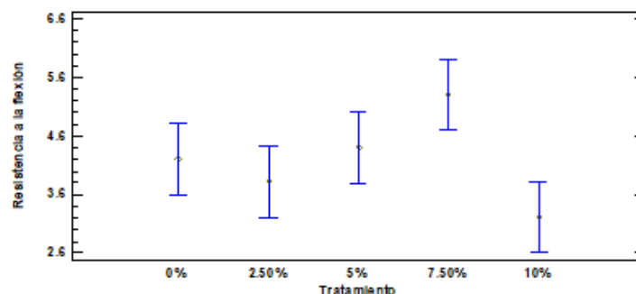
Figura 64 Gráfico de medias para Resistencia a la flexión a los 28 días.
