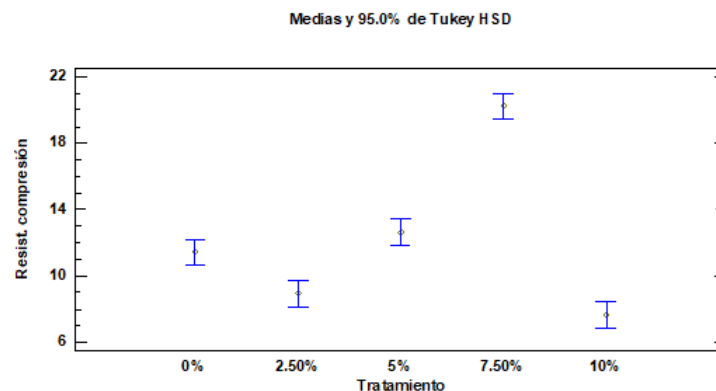
Figura 63 Gráfico de medias para Resistencia a la compresión a los 28 días adobe 25x13x10cm.
