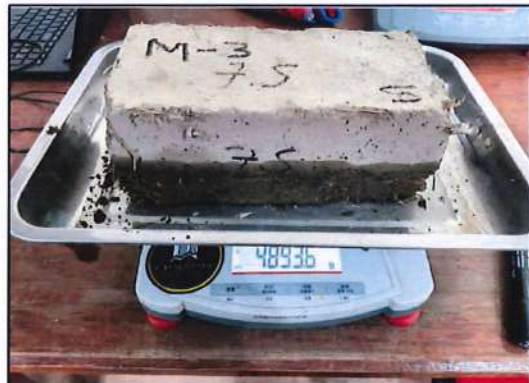
Figura 04: Peso de muestra saturada M-3 con 7.5% de ceniza de tallo de maíz
