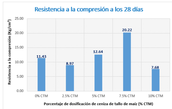
Figura 56 Resultados promedio del ensayo de la resistencia a la compresión (Kg/cm 2 ) de la unidad de 25x13x10cm a los 28 días.
