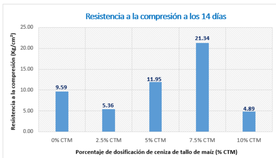
Figura 54 Resultados promedio del ensayo de la resistencia a la compresión (Kg/cm 2 ) a los 14 días.
