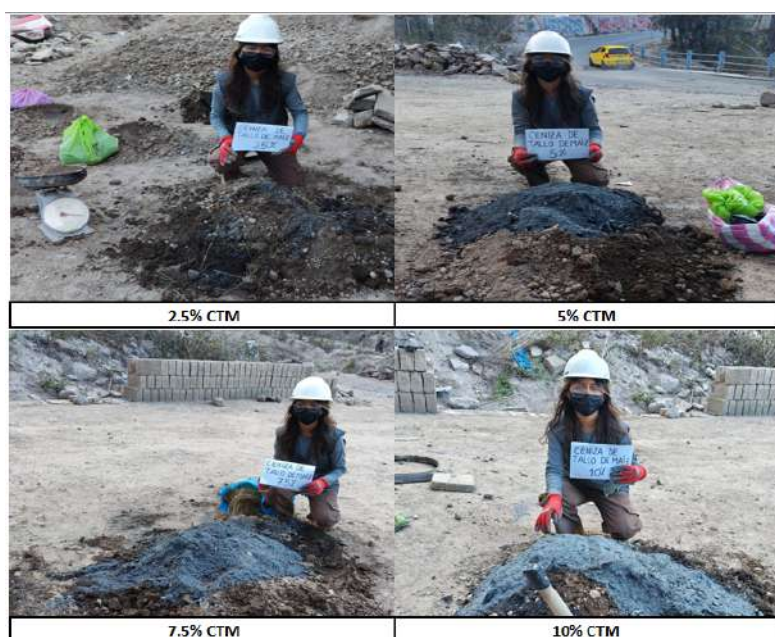
Figura 28 Formación de la masa de adobe con distintas dosificaciones.
