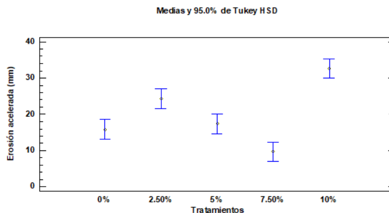
Figura 61 Gráfico de medias para Erosión acelerada (mm) por tratamientos.
