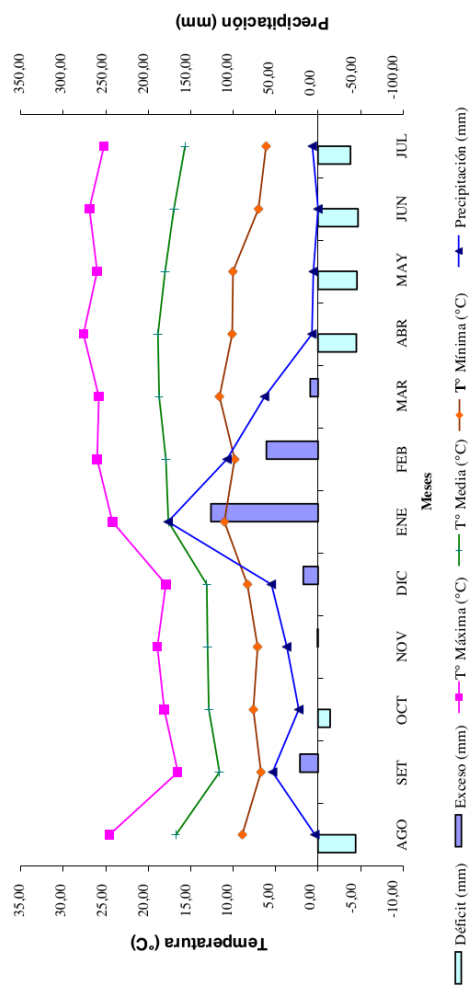
Figura 2.1. Temperaturas ombrotérmicas y balance hídrico, correspondiente a la campaña agrícola 2022 - 2023. Estación Meteorológica Canadán INIA - Ayacucho.
