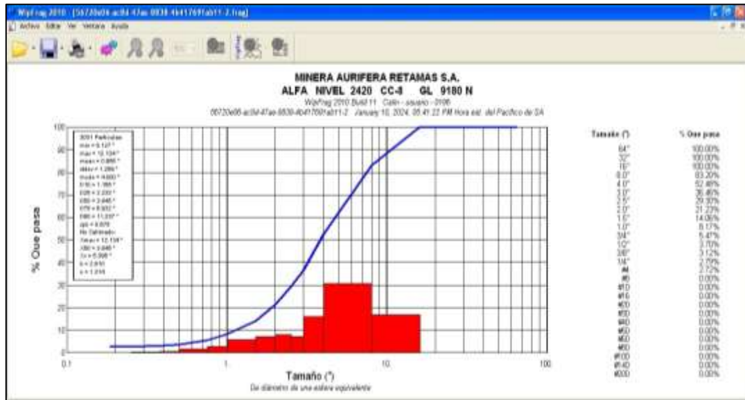
Figura 29. P80 del desmonte – 7.4”.
