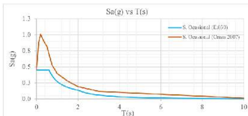
Fig. 91 Aceleración espectral para Sismo Ocasional.
