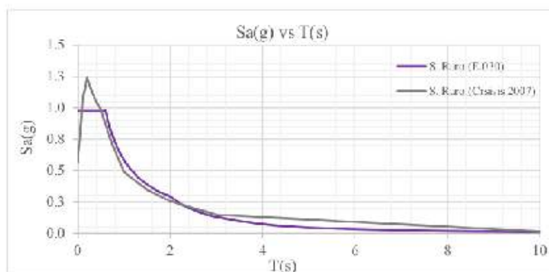
Fig. 92 Aceleración espectral para Sismo Raro.
