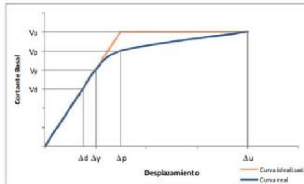
Fig. 63 Curva de capacidad, Ern-Capra.
