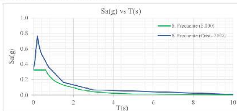
Fig. 90 Aceleración espectral para Sismo Frecuente.
