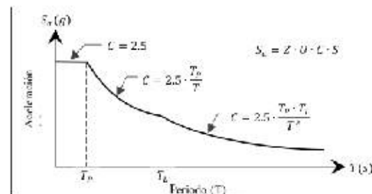
Fig. 79 Modelo de espectro según E.030
