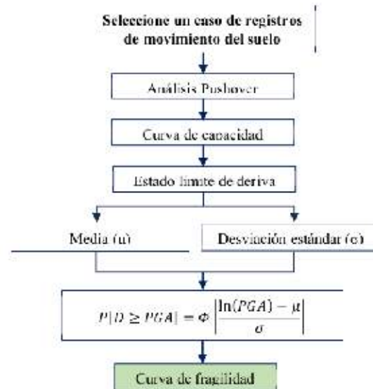
Fig. 59 Diagrama de flujo general del desarrollo de la curva de fragilidad según Mohamed, P.; et. al, 2017
