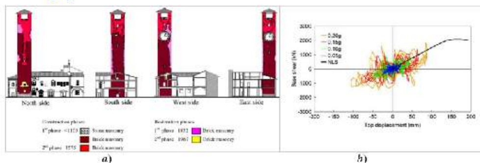
Fig. 25 Evaluación sísmica de una torre de mampostería histórica (Cremona Italia). a) Modelo matemático de la edificación y b) Resultados de la curva de histéresis.
