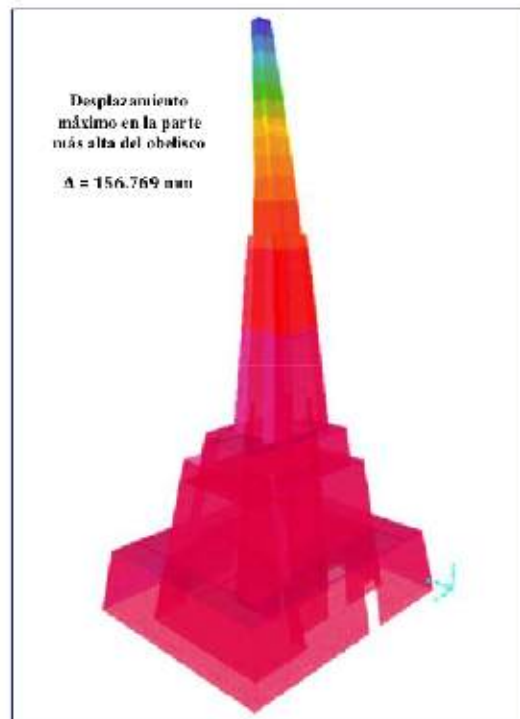
Fig. 102 Desplazamiento máximo en el nudo 73 del obelisco, SAP2000 25.1.0
