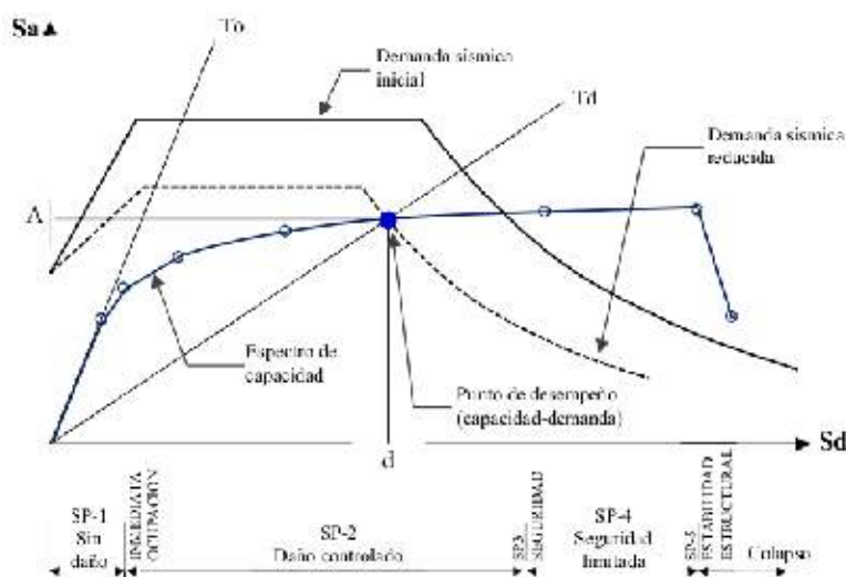
Fig. 39 Representación del método del espectro de capacidad.
