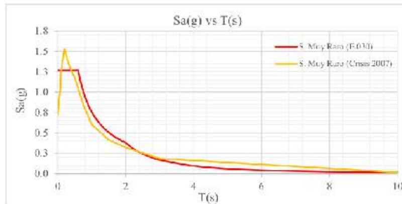
Fig. 93 Aceleración espectral para Sismo Muy Raro.
