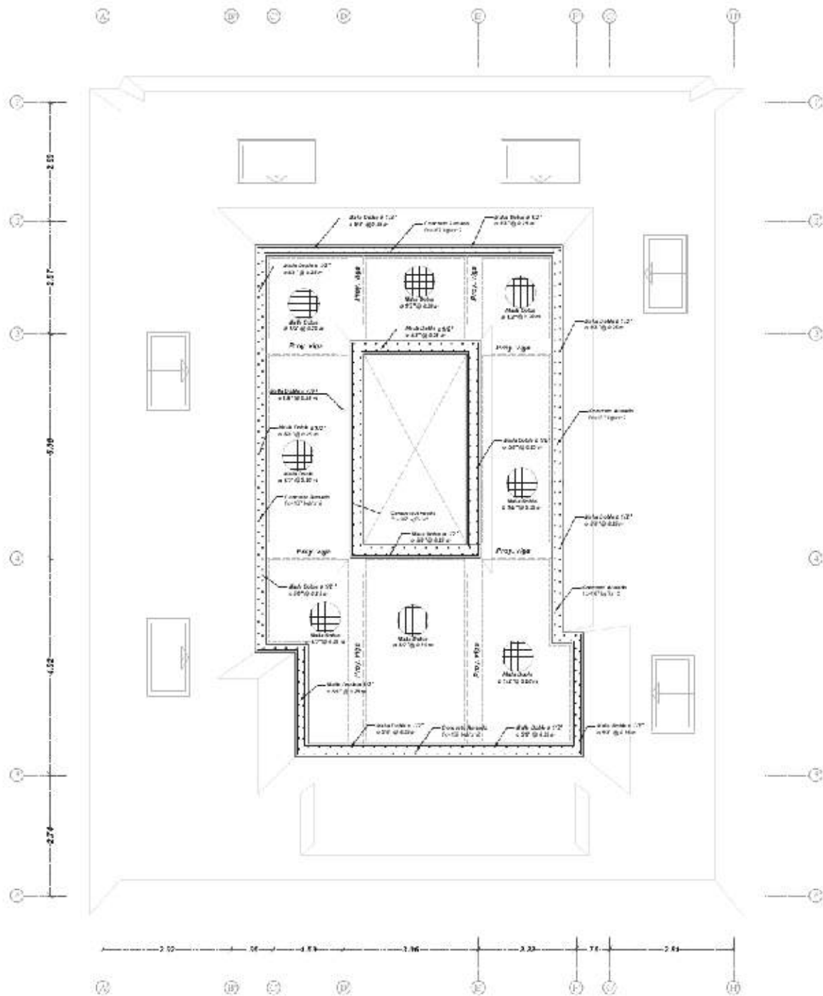
TERCER NIVEL Planta Esc. 1/100
