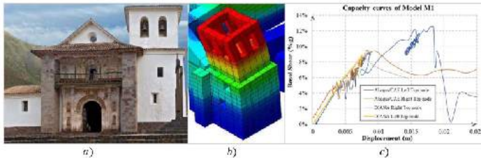
Fig. 26 Iglesia San Pedro apóstol de Andahuayllillas, Cusco. a) Templo de Andahuayllillas, b) Modelo tridimensional y c) Resultados.
