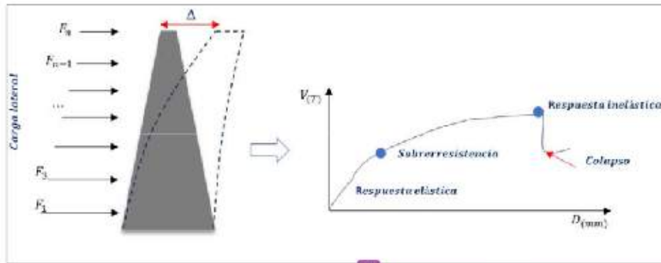
Fig. 33 Distribución de cargas laterales y la idealización del análisis Pushover según Arango, Paz y Duque, 2009.
