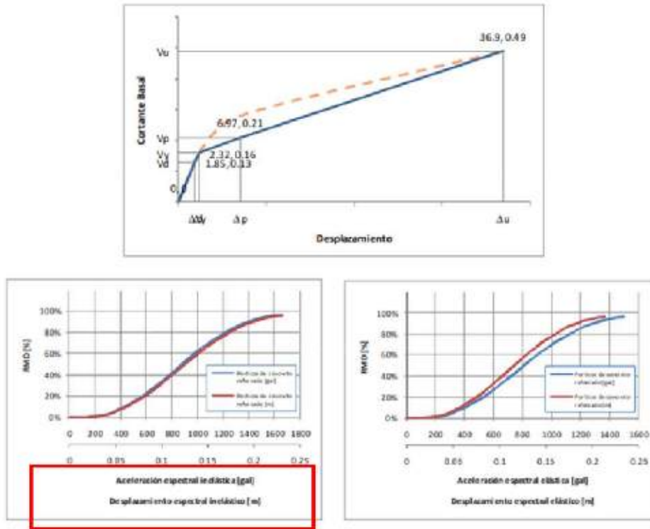
Fig. 66 Función de vulnerabilidad para diferentes variables, manual de Linn-Capra.
