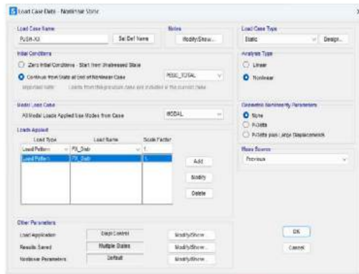
Fig. 85 Caso de carga no lineal estático.
