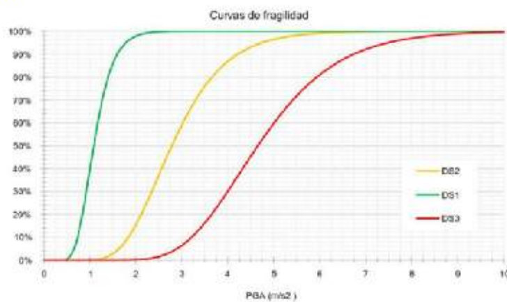
Fig. 67 Modelo de curva de fragilidad según programa FRACAS.
