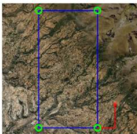
Fig. 51 Fuente generadora de 5x10 km.
