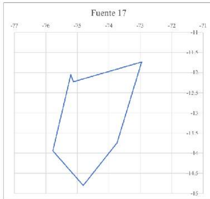
Fig. 47 Gráfico de la fuente 17.
