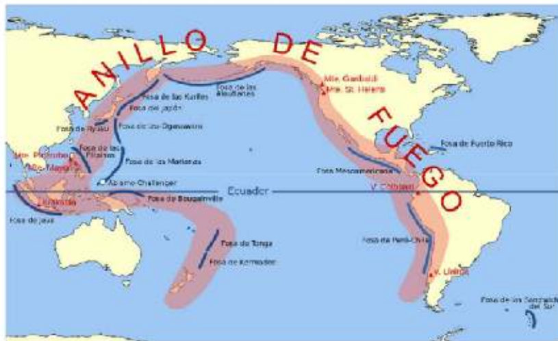
Fig. 1 Placas tectónicas pertenecientes al Anillo de Fuego [1].
