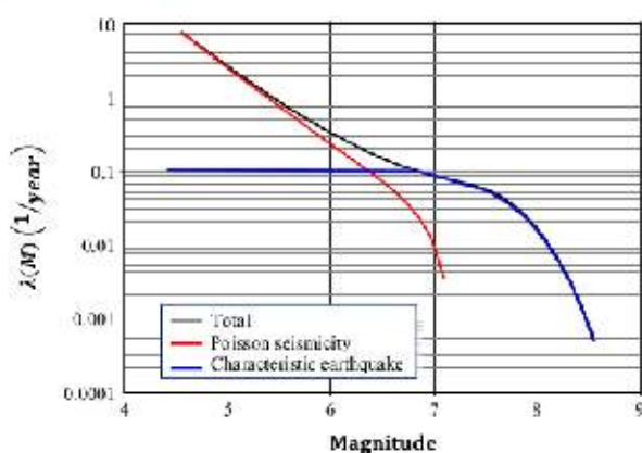
Fig. 73 Modelo de Gutenberg-Richter modificado.
