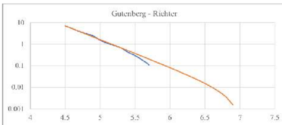
Fig. 49 Curva de Gutenberg & Richter.
