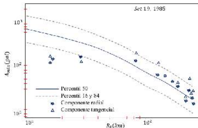
Fig. 41 GMPE del sismo de México, 19 de septiembre de 1985. diapositiva, Antonio Zevallos Cabrera, programa maestría PLICP, 2020.
