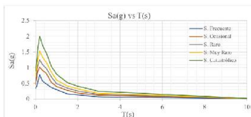
Fig. 88 Ordenada espectral para diferentes periodos de retorno.
