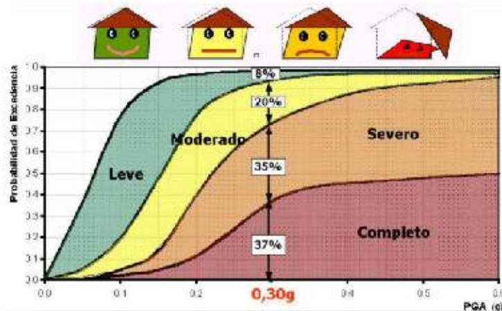
Fig. 61 Ejemplo de Curvas de fragilidad en función de PGA según Velásquez, 2006.
