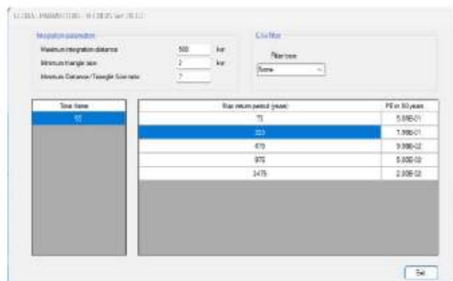
Fig. 77 Matriz de consideración para sismos con diferentes periodos de retorno.
