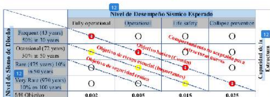
Fig. 35 Niveles de desempeño sísmico esperado según el comité de Visión 2000 del SEAOC 1993.
