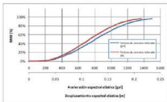
Fig. 62 Función de vulnerabilidad para pórticos de concreto y para diferentes intensidades, Em Capra.
