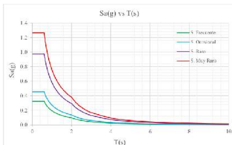
Fig. 89 Aceleración espectral según E.030
