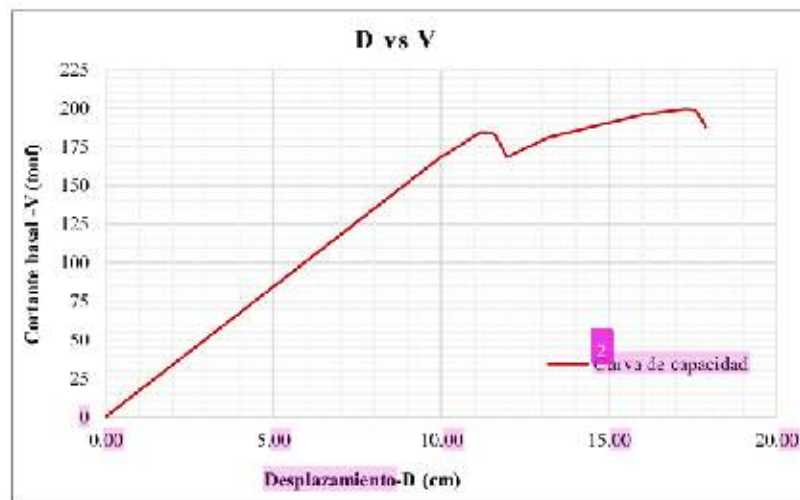
Fig. 94 Curva Pushover del obelisco sin reforzamiento.
