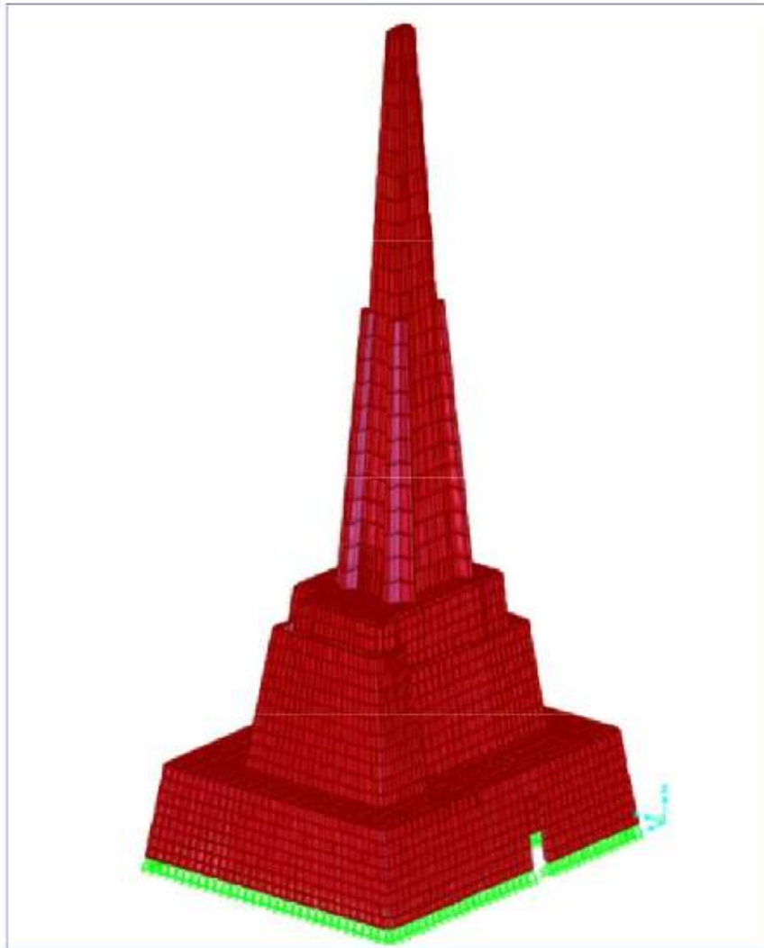
Fig. 81 Modelo de elementos finitos (3D).
