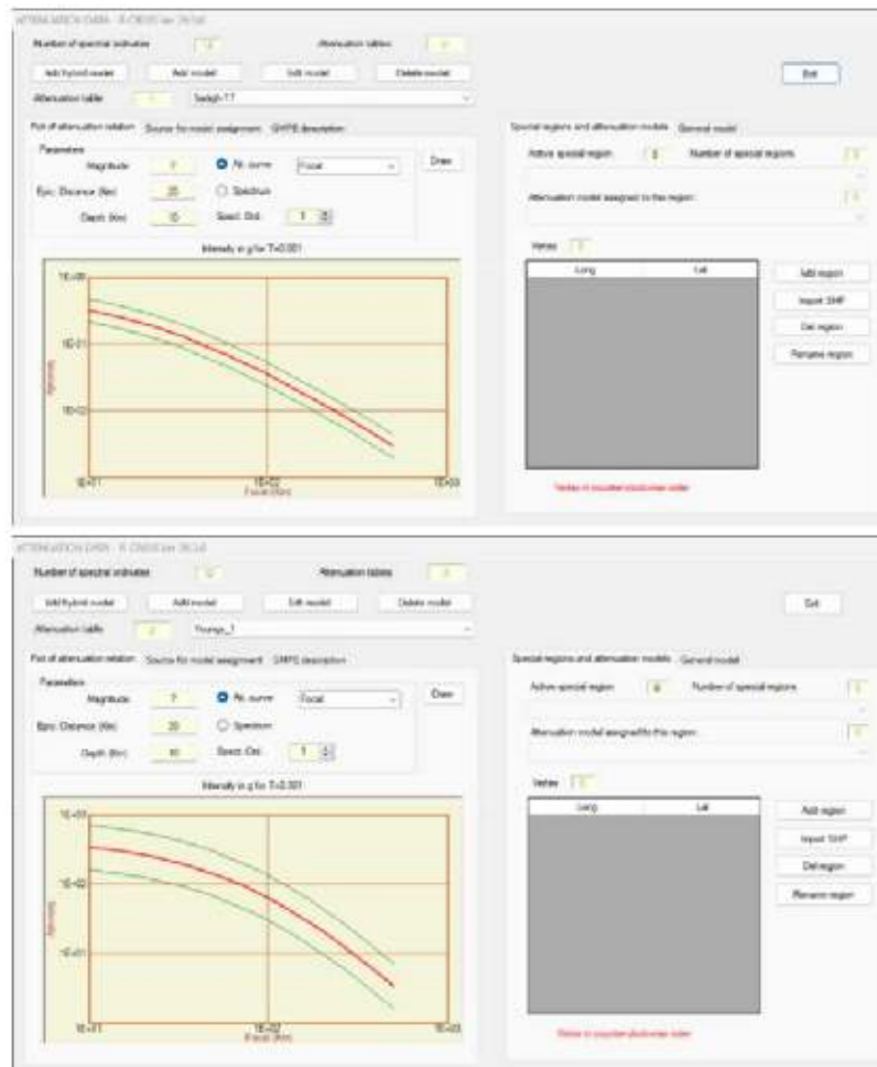
Fig. 75 Leyes de atenuación de Sadigh y Young
