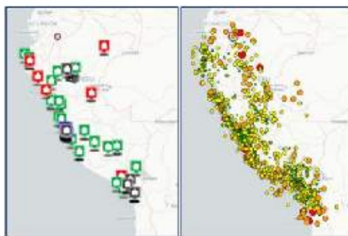
Fig. 68 Sismología activa en Perú.
