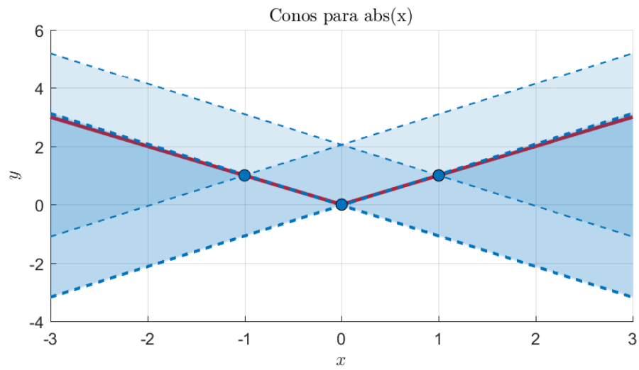
Figura 2.14: Conos C(\mathbf{x}_0; L) de f(x) = |x| , para \mathbf{x}_0 = -1, 0, 1 .
