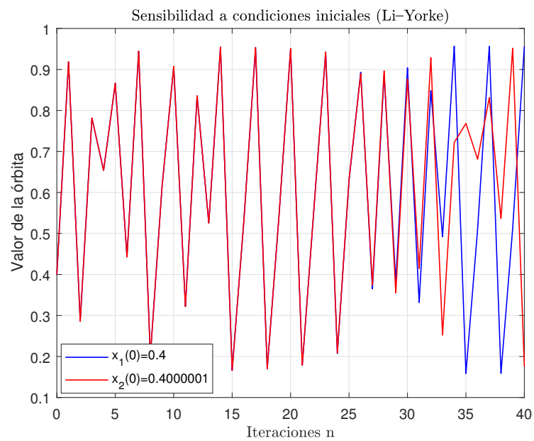
Figura 2.21: Órbitas f^n(x_1) y f^n(x_2) para n = 0, 1, \dots, 40
