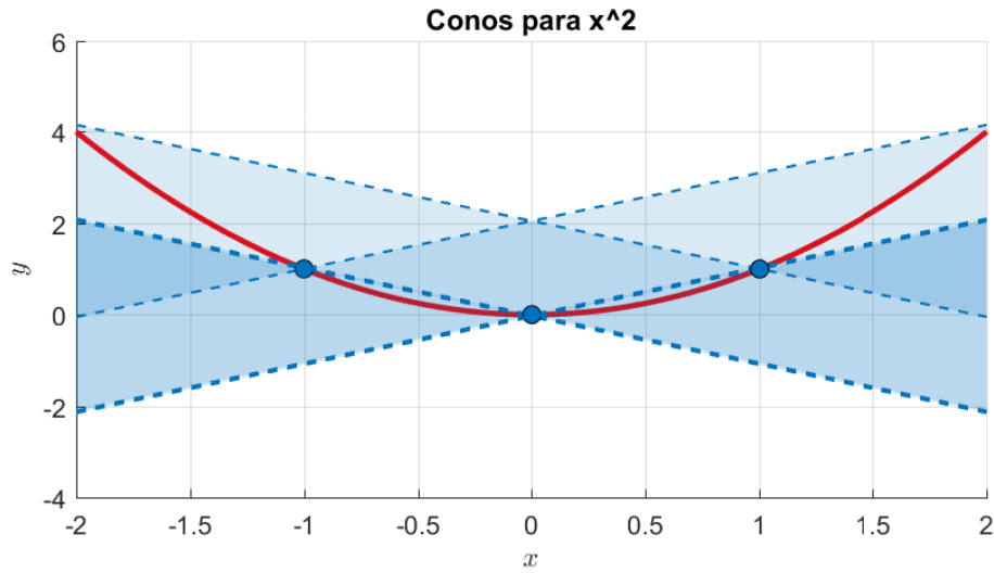
Figura 2.13: Conos C(\mathbf{x}_0; L) de f(x) = x^2 , para \mathbf{x}_0 = -1, 0, 1 .
