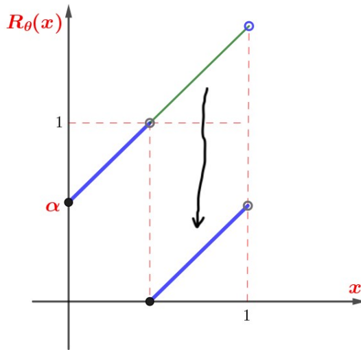
Figura 2.4: Rotación R_\theta .
