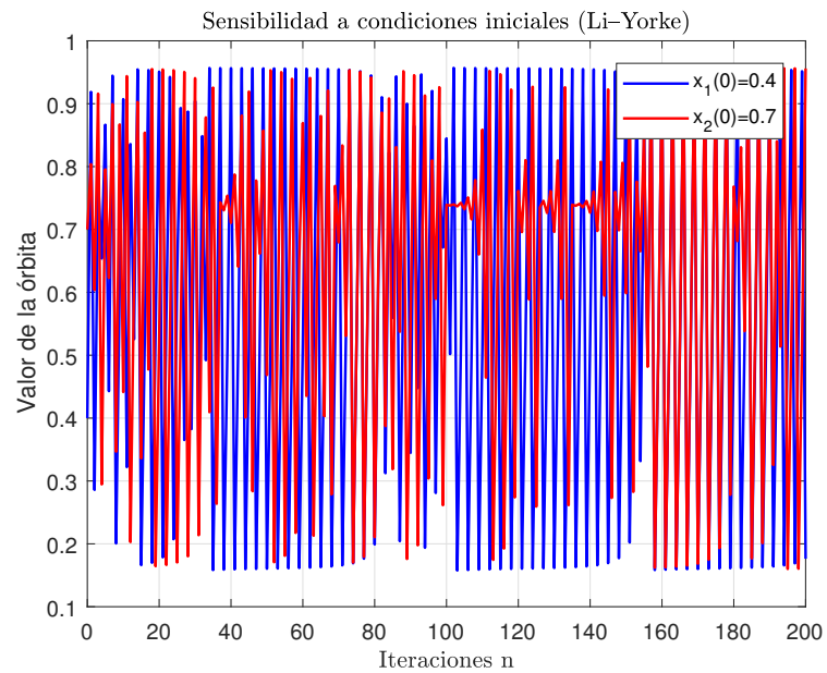
Figura 2.20: Órbitas f^n(x_1) y f^n(x_2) para n = 0, 1, \dots, 200
