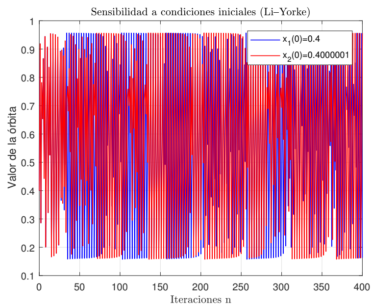
Figura 2.22: Órbitas f^n(x_i) , i = 1, 2 y para n = 0, 1, \dots, 400
