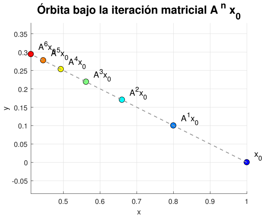
Figura 2.11: Órbitas \mathbf{A}^n \mathbf{x}_0 , para n = 6 .
