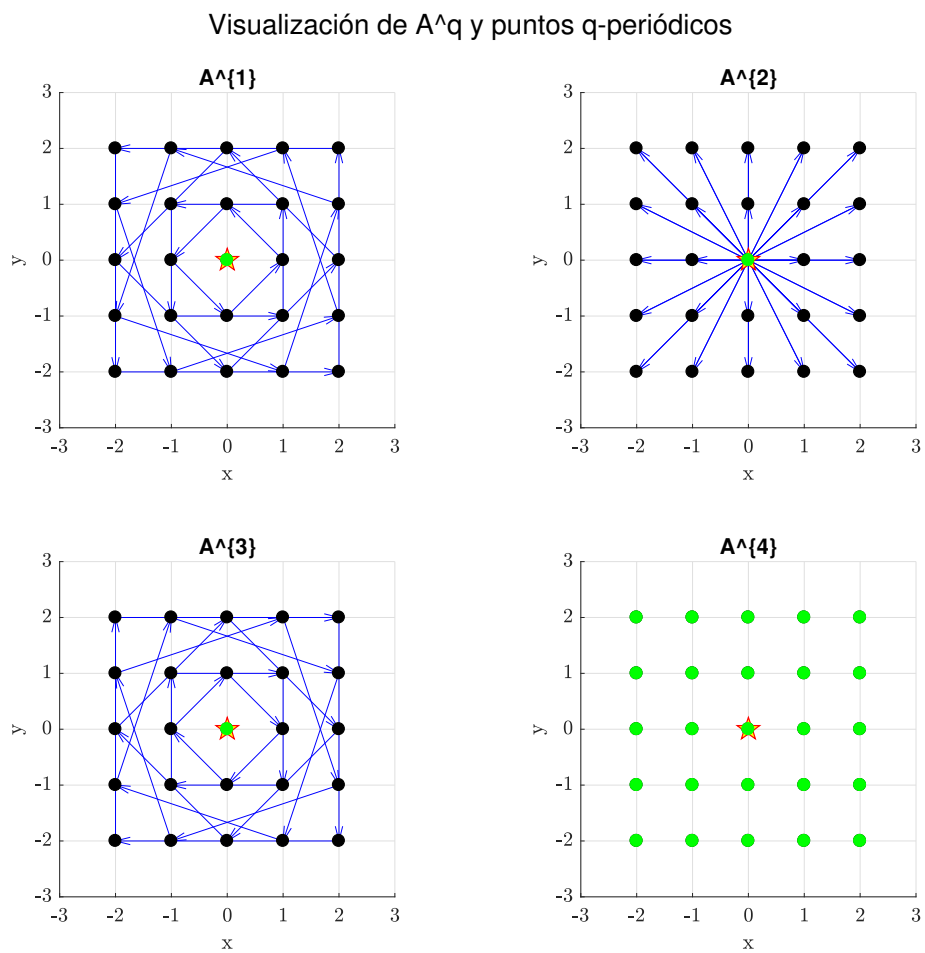
Figura 2.8: Puntos q -periódicos.
