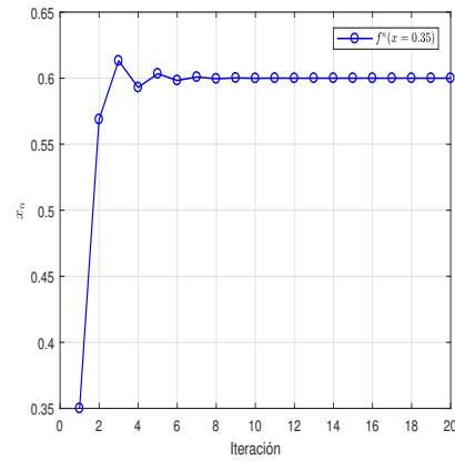
Figura 4.2: Órbitas f_{2.5}^n(x) , n = 1, 2, \dots, 20 .
