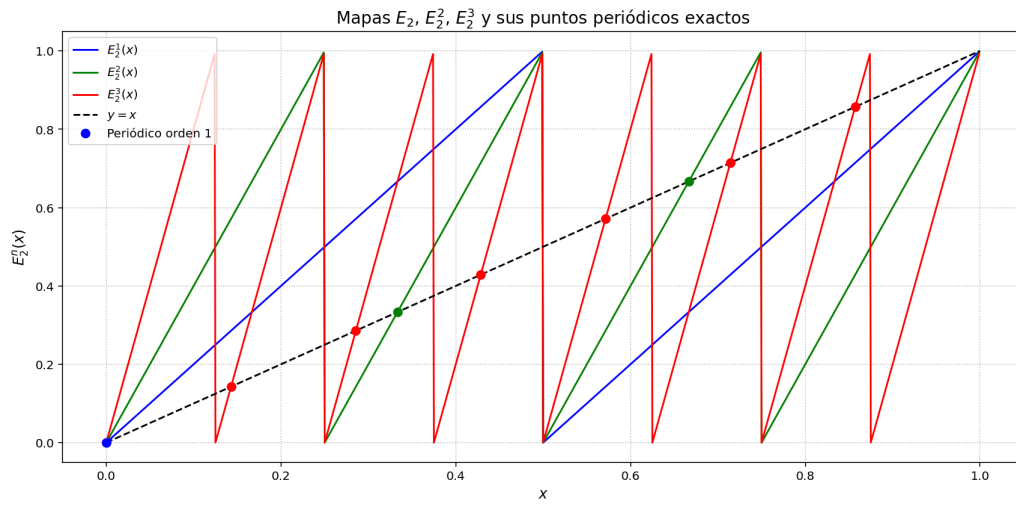
Figura 2.7: E_2 , E_2^2 y E_2^3 junto con sus puntos q -periódicos (azul: orden q = 1 , verde: orden q = 2 , rojo: orden q = 3 ).
