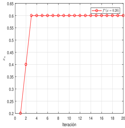
Figura 4.2: Órbitas f_{2.5}^n(x) , n = 1, 2, \dots, 20 .
