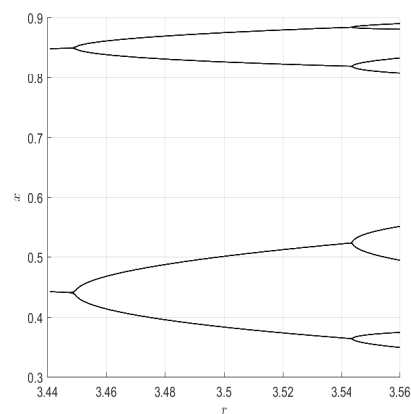
(d) 3.441 \leq r \leq 3.56 .
