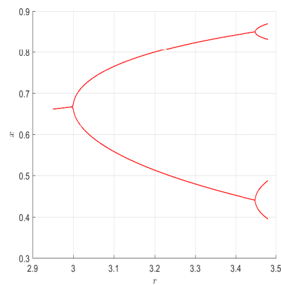
Figura 4.3: Diagrama de bifurcación del mapa logístico.
