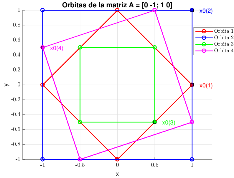
Figura 2.9: Puntos q -periódicos.
