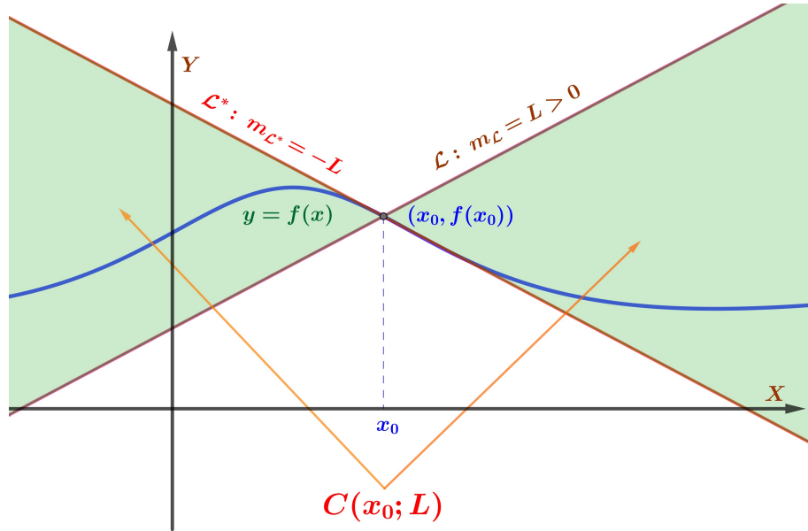
Figura 2.12: Cono C(\mathbf{x}_0; L) .
