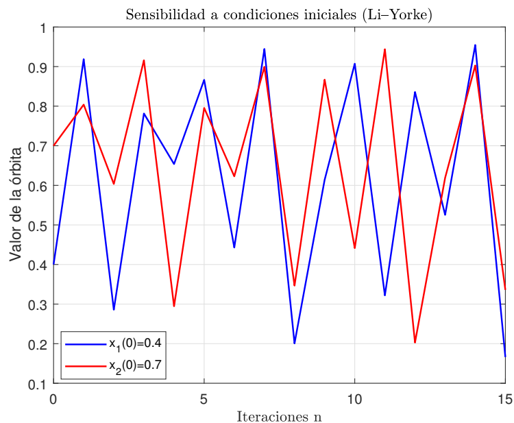
Figura 2.19: Órbitas f^n(x_1) y f^n(x_2) para n = 0, 1, \dots, 15
