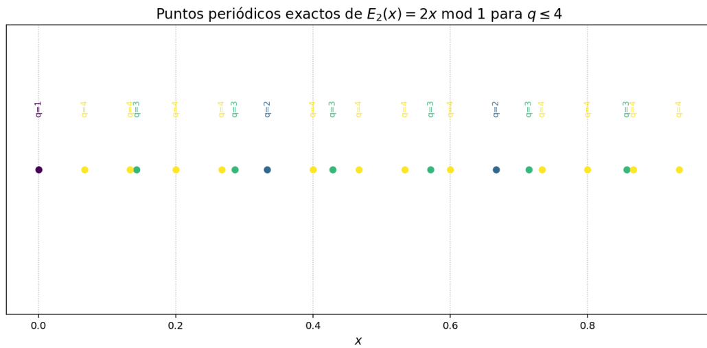
Figura 2.6: Puntos periódicos de E_2 de orden q \leq 4 .
