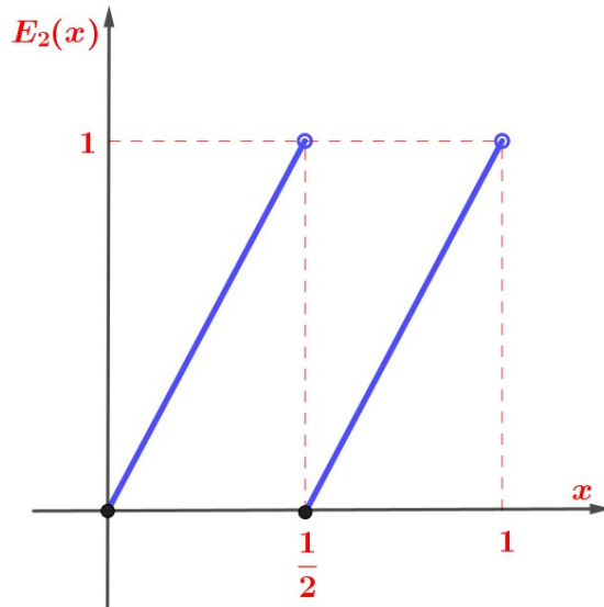
Figura 2.5: Aplicación E_2(x) .
