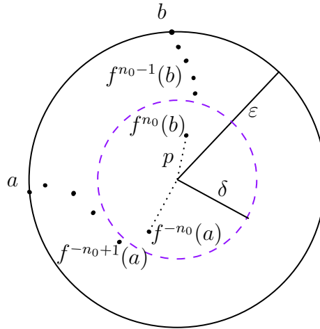
Figura 2.1: f^n b \rightarrow p y f^{-n}(a) \rightarrow p cuando n \rightarrow \infty , .
