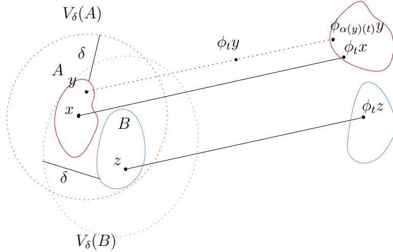
Figura 3.1: Hiper-expansividad
