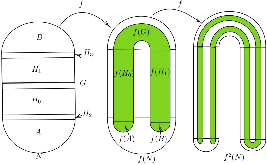
Figura 1.4: La herradura de Smale
