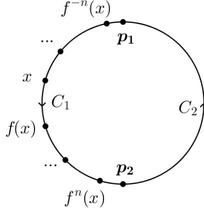
Figura 1.3: S^1
