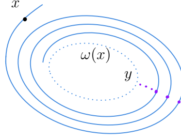
Figura 1.1: Conjunto Omega limite \omega(x)
