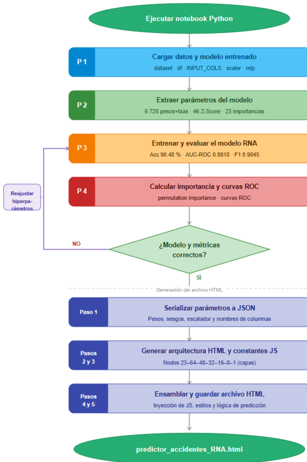
Figura 120 Diagrama de flujo de la creación del programa RNA N°01
