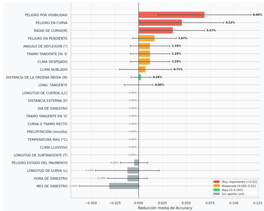
Figura 116 Reducción media de Accuracy por variable (promedio ± desviación estándar, 20 repeticiones)
