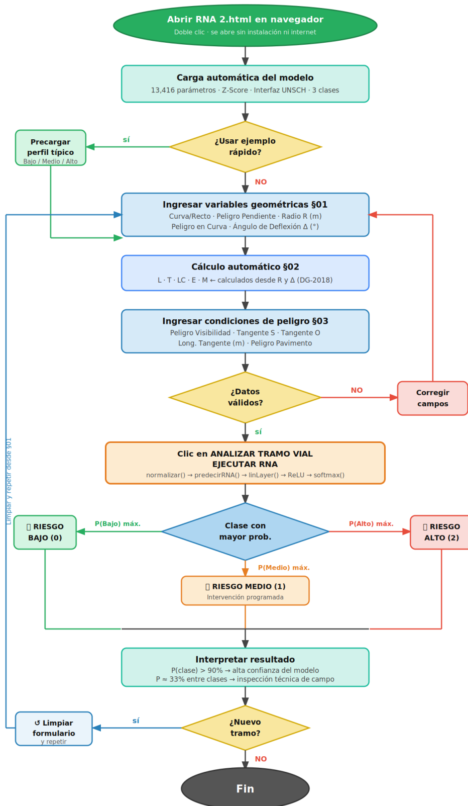
Figura 190 Diagram de flujo de uso del programa RNA N°02
