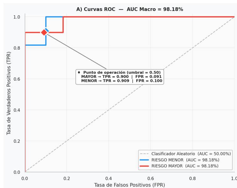
Figura 211 Curva ROC y área bajo la curva (AUC) del modelo RNA. Fuente: Elaboración propia
