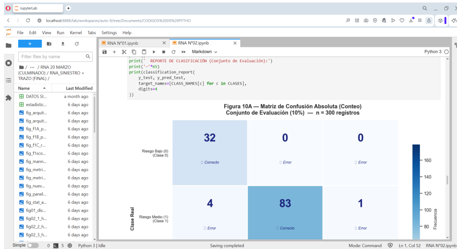
Figura 272 Matriz de confusión. Fuente: Elaboración propia
