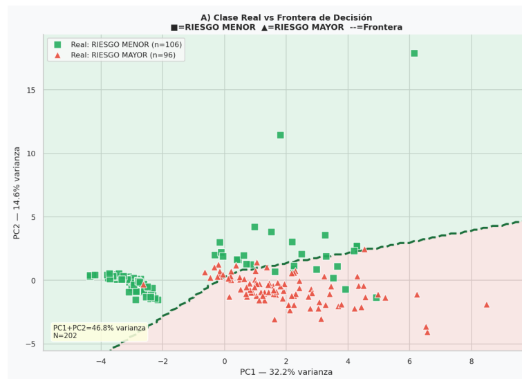
Figura 210 Clase Real vs Frontera de Decisión. Fuente: Elaboración propia
