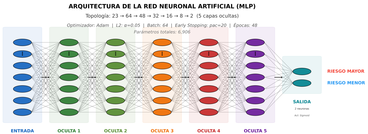
Figura 208 Arquitectura del Perceptrón Multicapa de la RNA N°01
