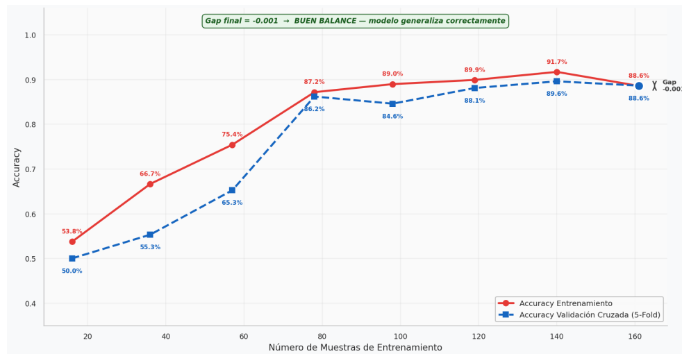
Figura 113 Curva de Aprendizaje: Diagnóstico de Sobreajuste.
