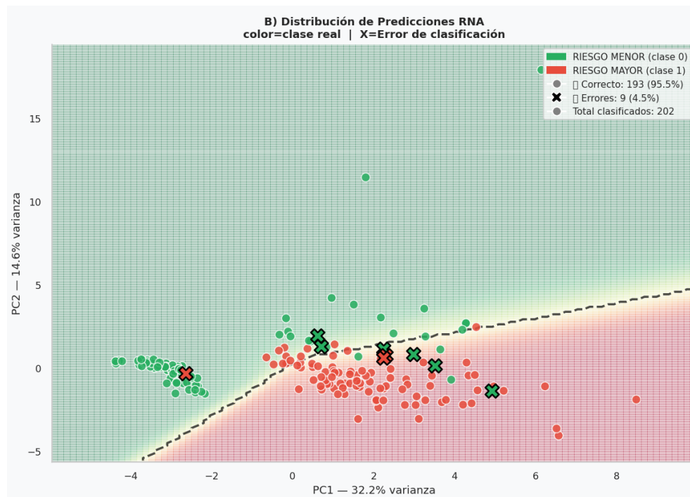
Figura 115 Distribución de Predicciones y Confianza del Modelo.
