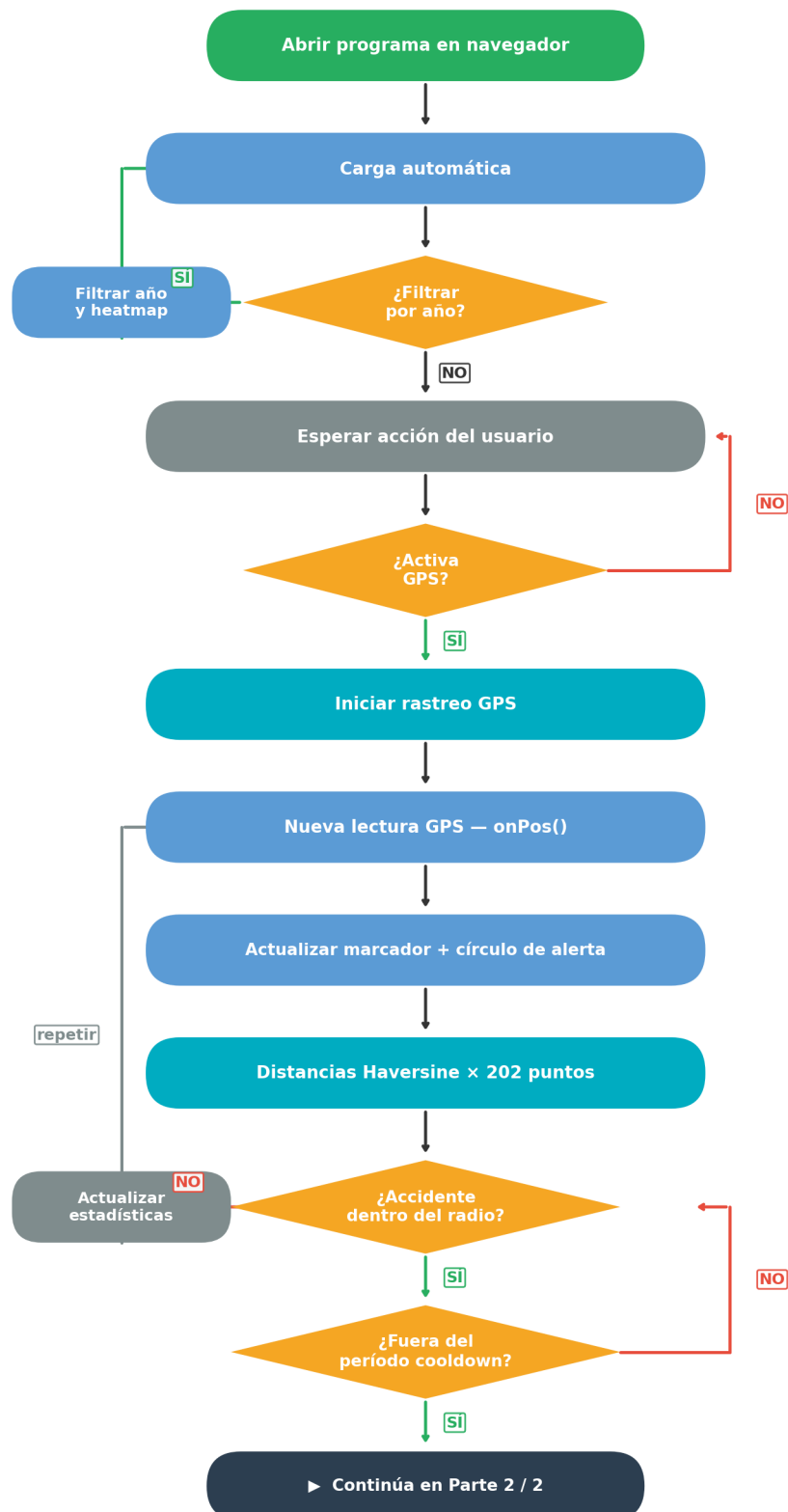
Figura 197 Diagrama de flujo - Parte I.
