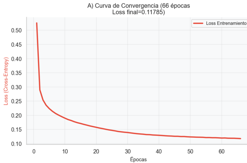
Figura 172 Curva de convergencia.
