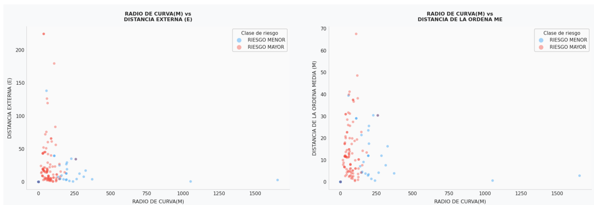
Figura 85 Diagr. de disper. Radio de curva vs Dist. Externa vs Dist. de la ord. media. Fuente: Elaboración propia
