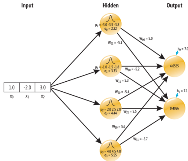
Figura 22 Redes neuronales de Base Radial
