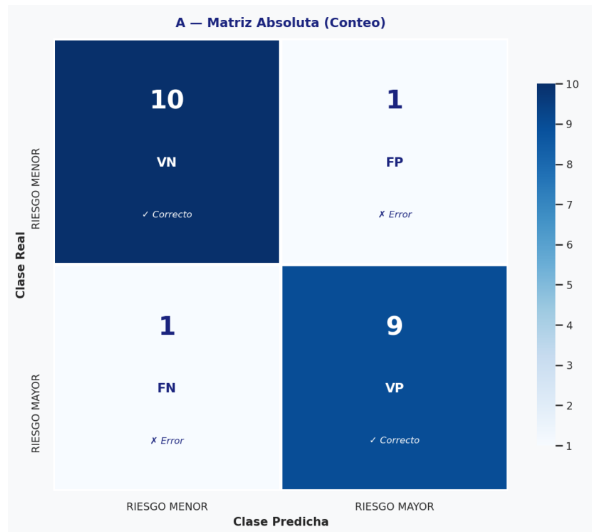
Figura 108 Matriz de Confusión del Modelo.
