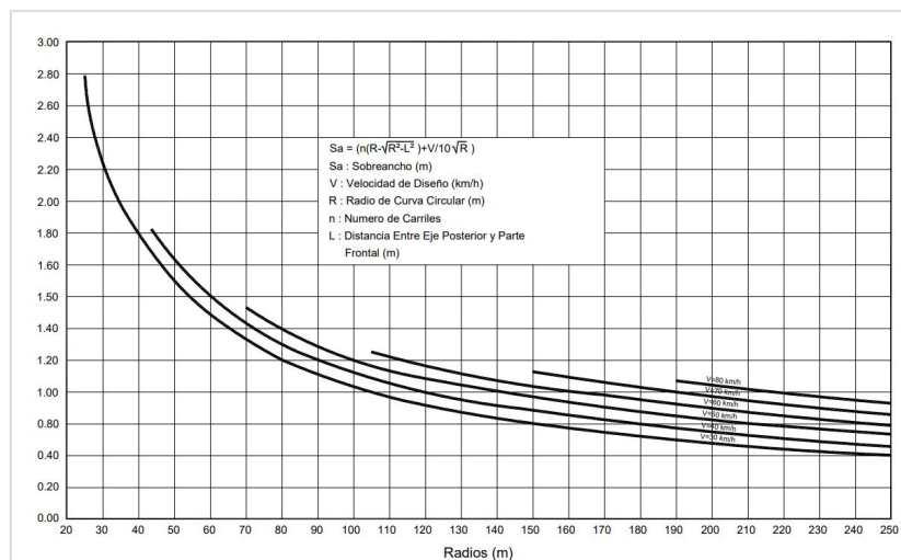
Figura 47 Valores de sobreancho en función a “L” del tipo de vehículo de diseño
