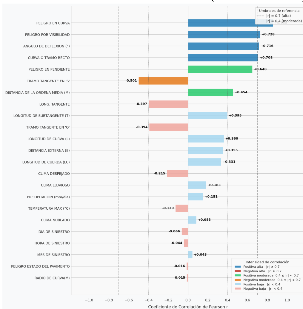
Figura 77 Barras de correlación individual con la variable objetivo
