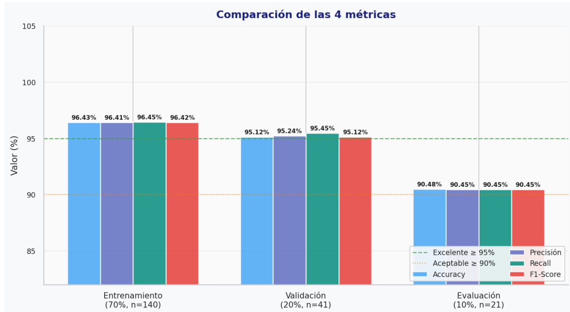
Figura 209 Comparación de las 4 métricas por partición.
