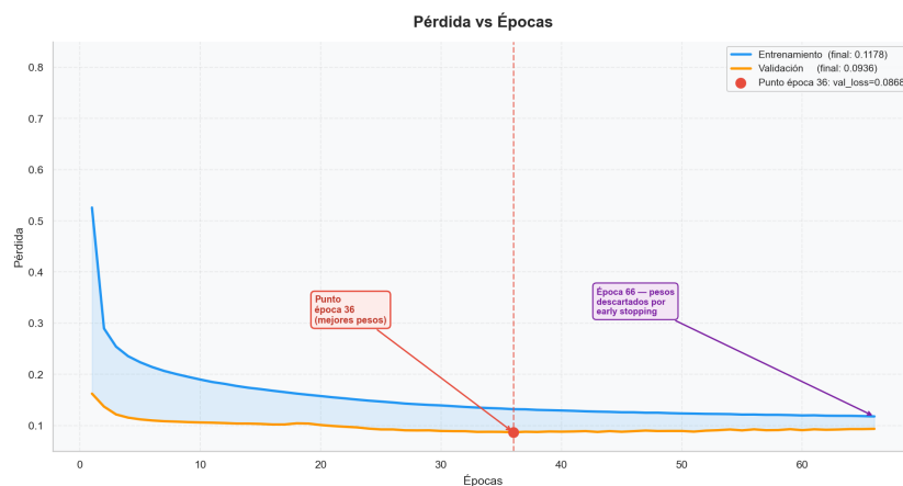
Figura 221 Pérdida vs épocas. Fuente: Elaboración propia
