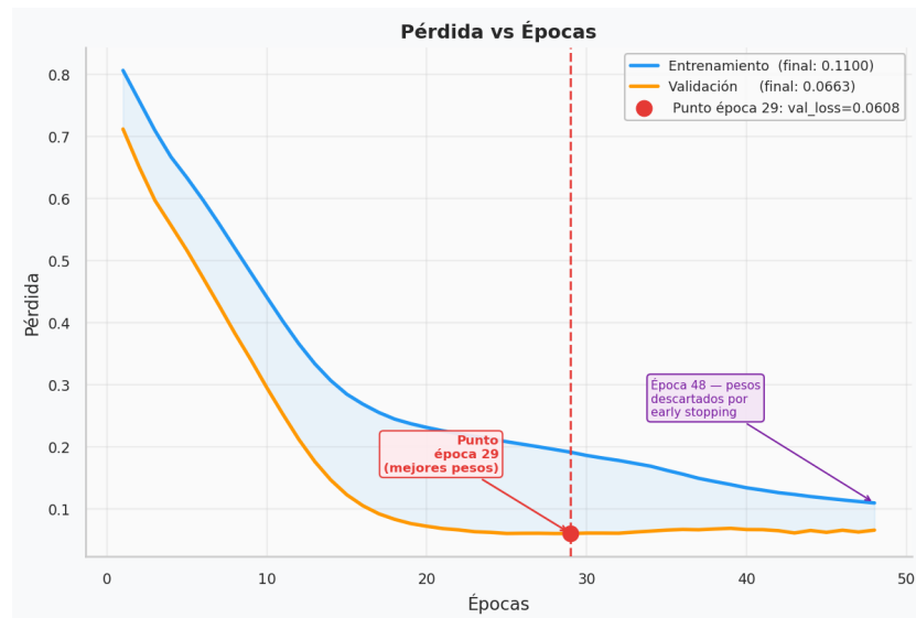
Figura 212 Pérdida (loss) vs. Épocas
