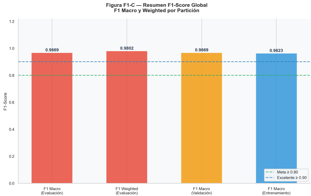
Figura 178 F1-Score global. Fuente: Elaboración propia
