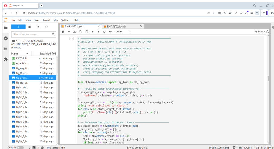
Figura 247 Arquitectura de la RNA N°01.
