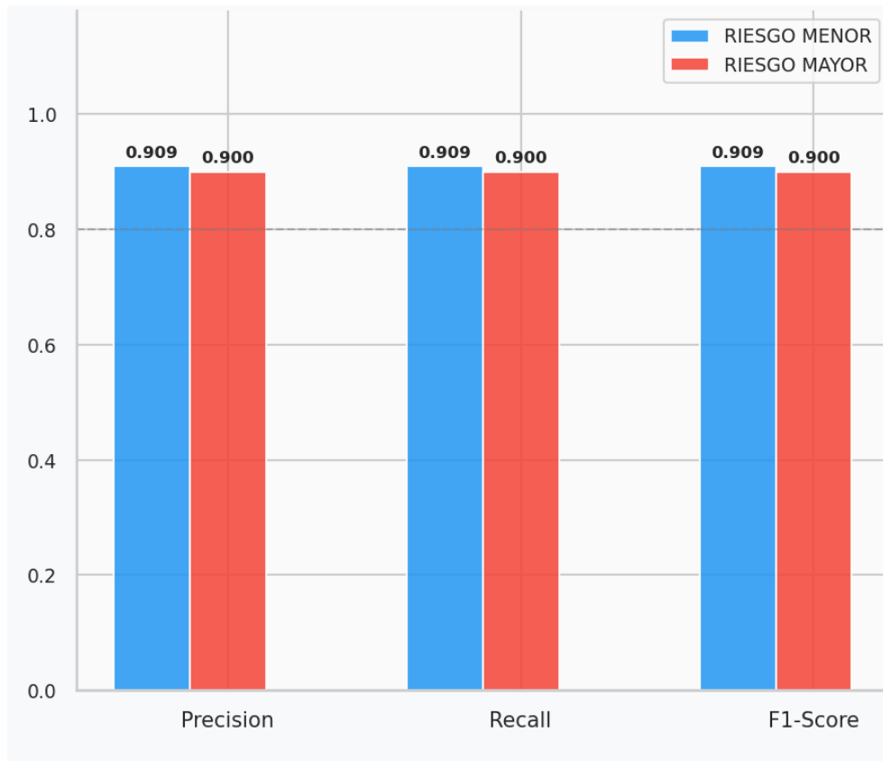
Figura 106 Precisión, Recall y F1-Score por Clase.
