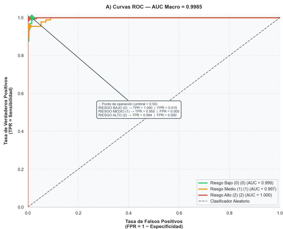
Figura 220 Curvas ROC y área bajo la curva (AUC).
