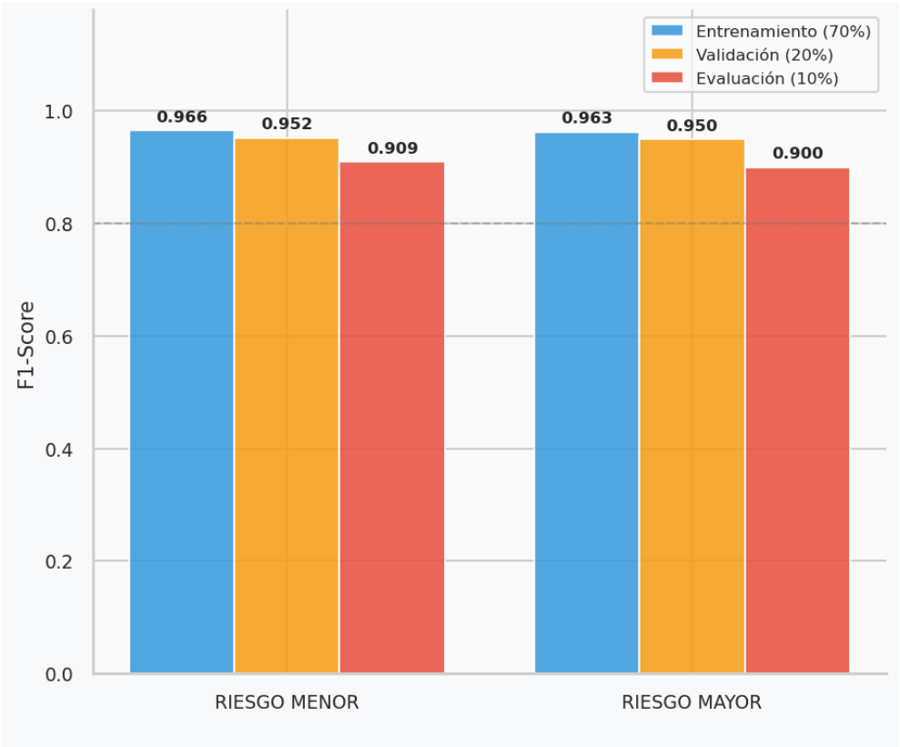
Figura 105 F1-Score por Clase en las Tres Particiones. Fuente: Elaboración propia
