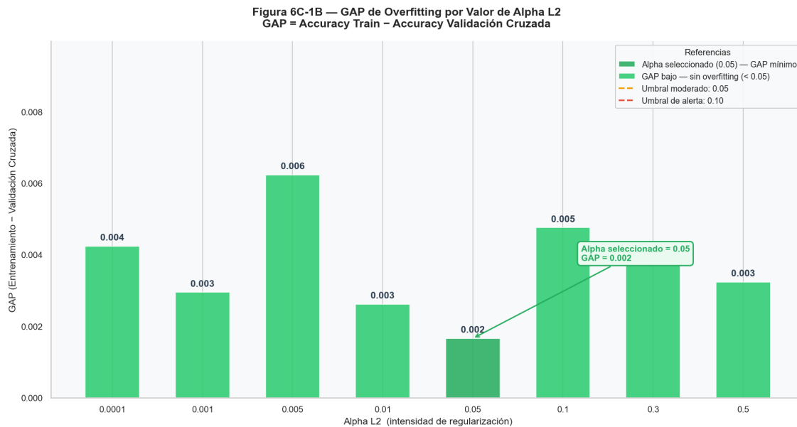
Figura 168 GAP vs Alfa L2.
