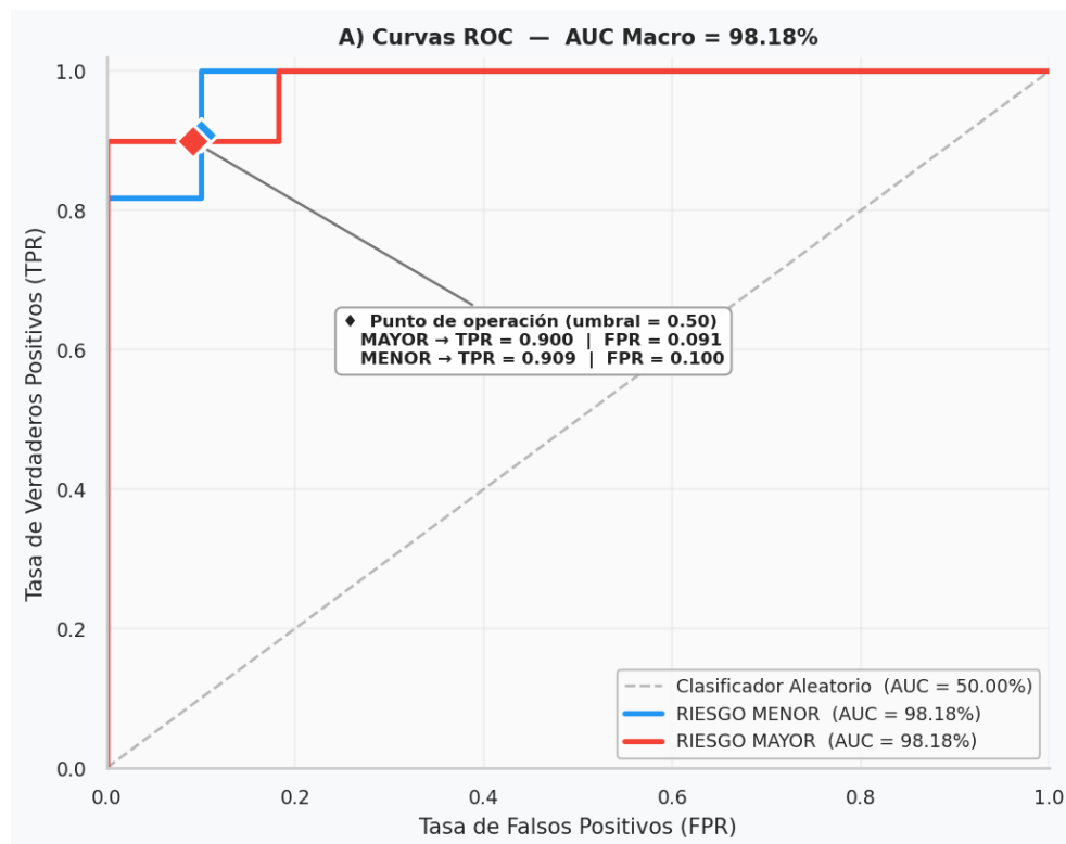
Figura 112 Curva ROC y área bajo la curva (AUC) del modelo RNA.
