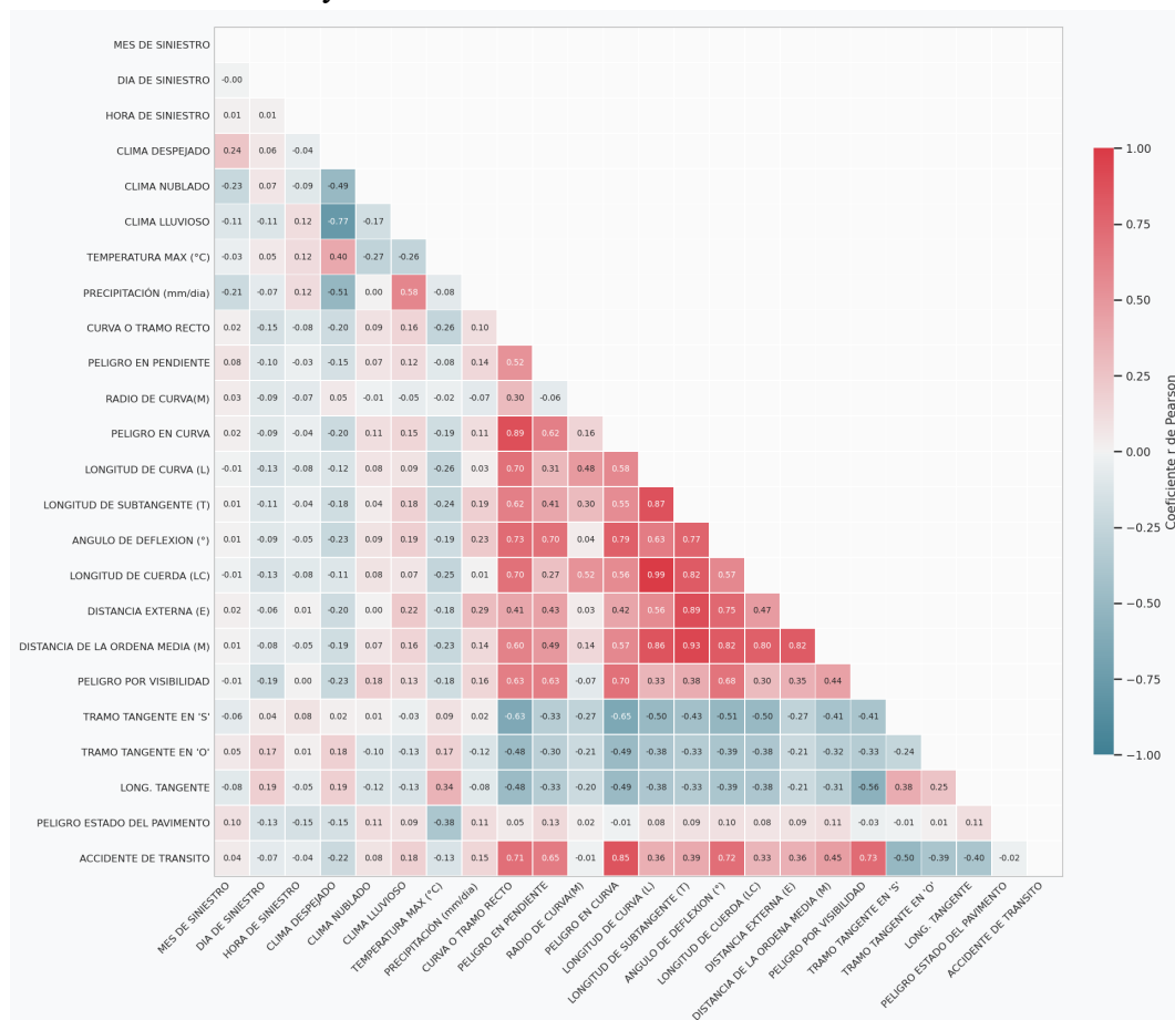
Figura 76 Heatmap de correlaciones de Pearson entre las 23 variables de entrada.
