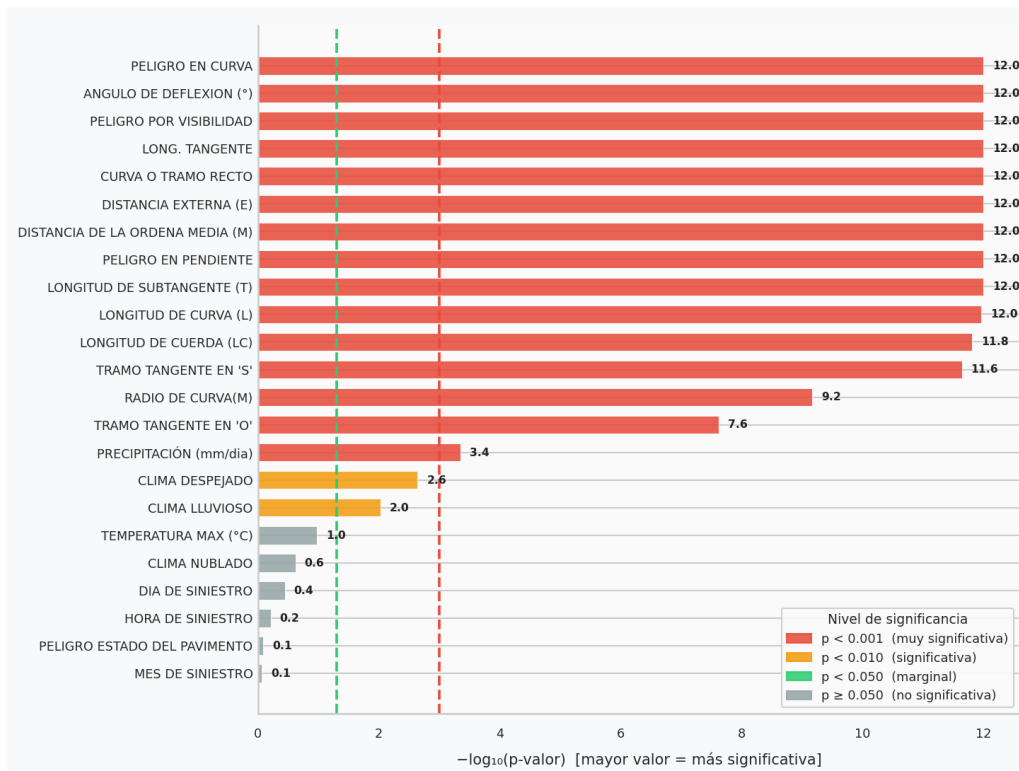
Figura 82 Análisis estadístico Mann-Whitney U de las 23 variables
