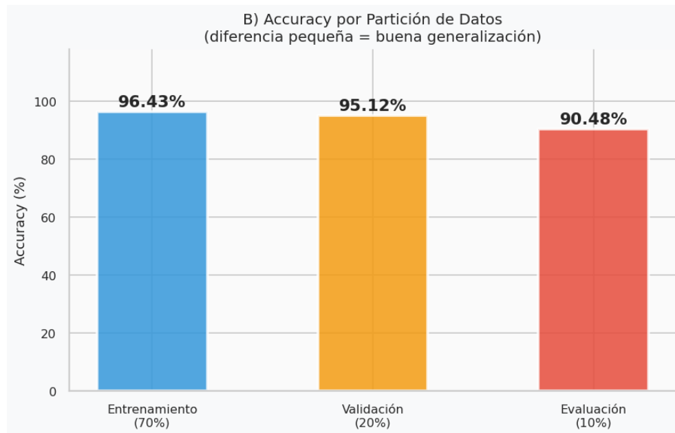
Figura 102 Accuracy en entrenamiento, validación y evaluación.
