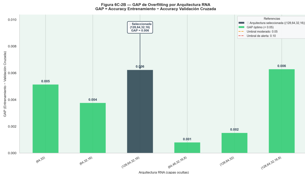
Figura 170 GAP vs por arquitectura de la RNA.
