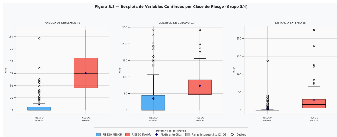
Figura 73 Boxplots de variables: Angulo de deflexión, Long. de cuerda y Dist. externa (E). Fuente: Elaboración propia
