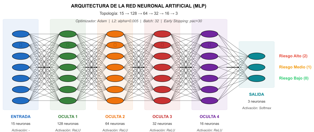
Figura 166 Arquitectura de la red neuronal N°02: 15 \rightarrow 128 \rightarrow 64 \rightarrow 32 \rightarrow 16 \rightarrow 3 . Optimizador Adam · L2 \alpha=0.05 Batch=32 Epocas=66.
