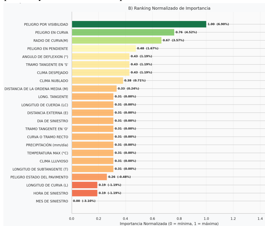
Figura 117 Ranking normalizado de importancia de variable
