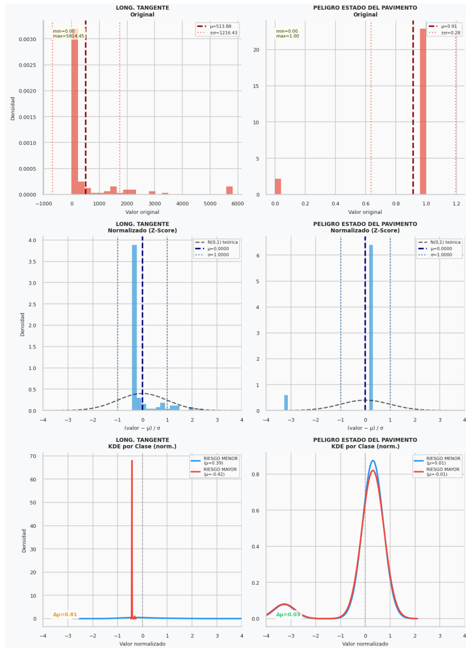
Figura 94 Normaliz. Z-Score: Longitud Tangente y Peligro Estado del Pavimento.
