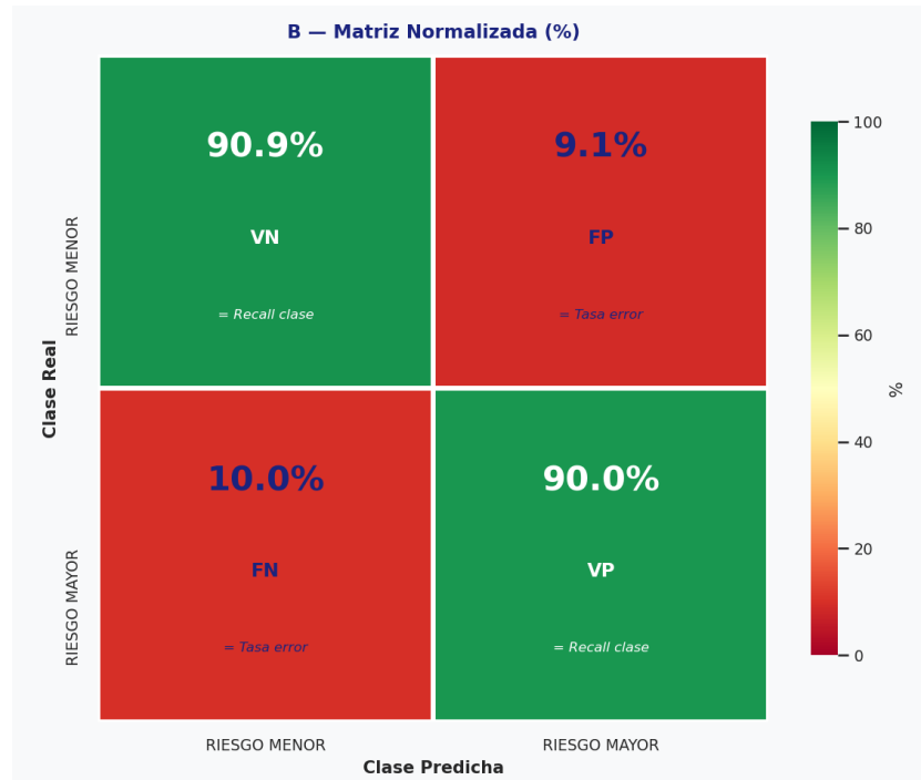
Figura 109 Matriz de confusión normalizada (%).
