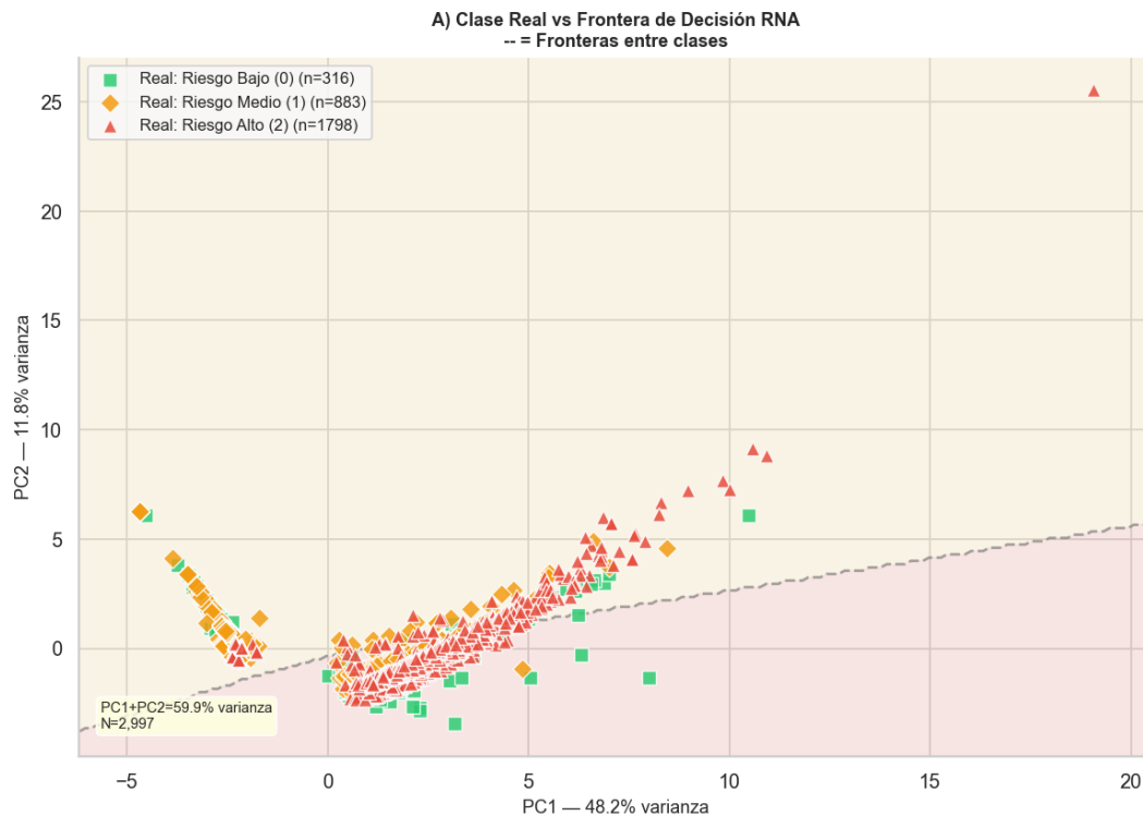
Figura 186 Clase real vs frontera de decisión del RNA.
