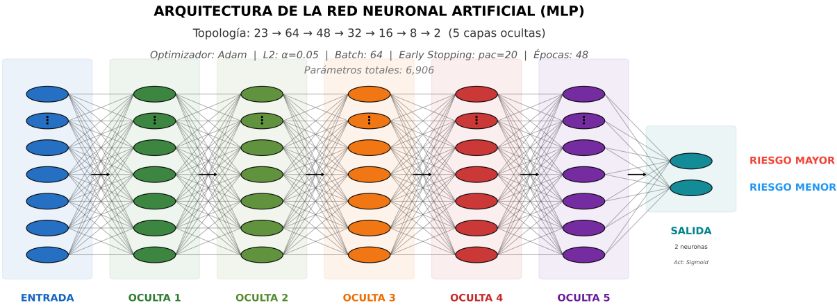
Figura 95 Arquitectura del Perceptrón Multicapa de la RNA N°01
