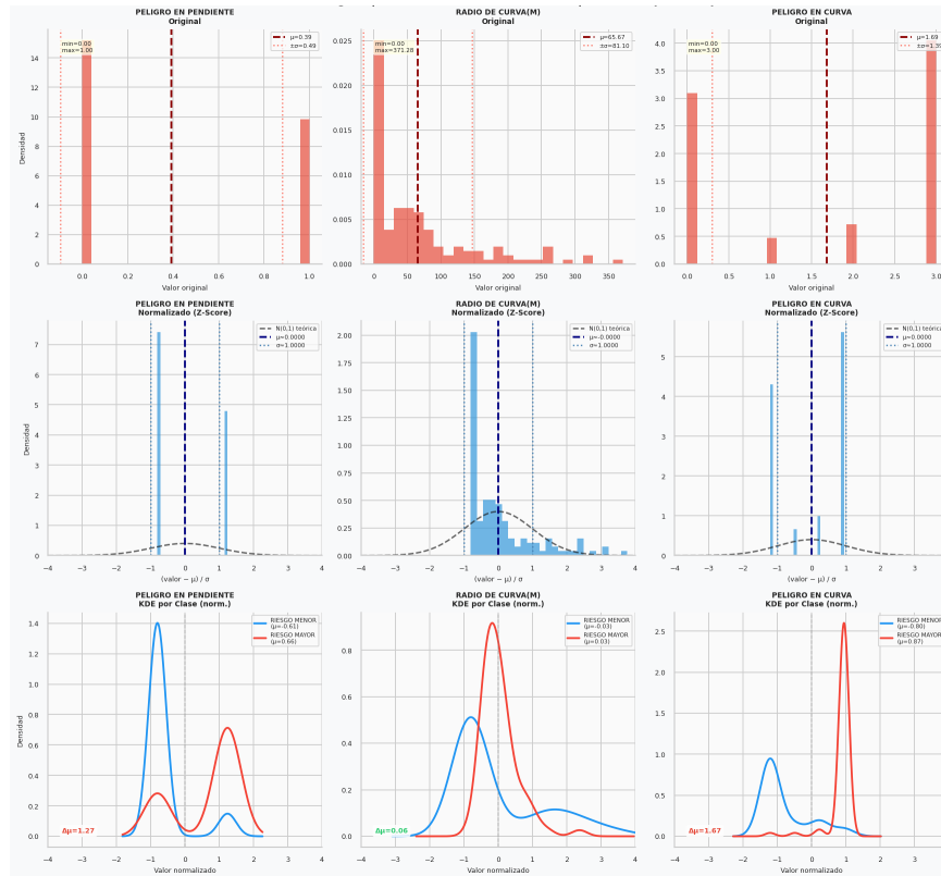
Figura 90 Normaliz. Z-Score: Peligro Pendiente, Radio de Curva y Peligro en Curva. Fuente: Elaboración propia
