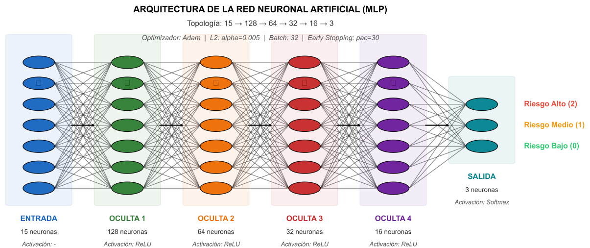
Figura 217 Arquitectura de la red neuronal N°02: 15 \rightarrow 128 \rightarrow 64 \rightarrow 32 \rightarrow 16 \rightarrow 3 . Optimizador Adam · L2 \alpha=0.005 Batch=32 Epocas=66.
