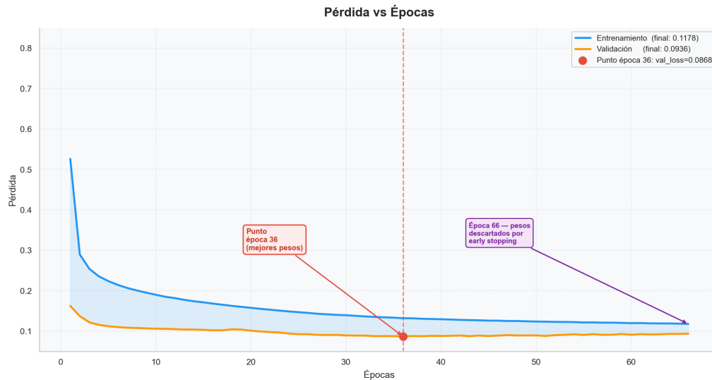
Figura 174 Pérdida vs épocas.
