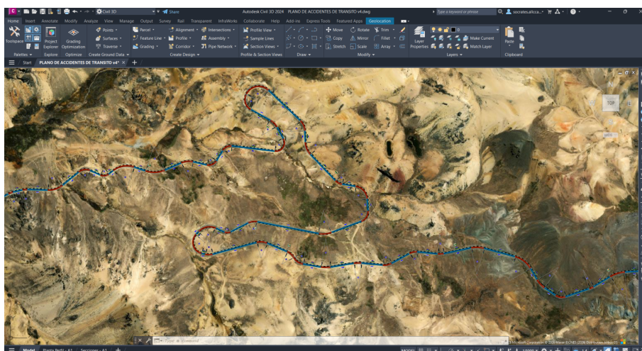
Figura 134 Modelamiento en el Civil 3D: Tramo Pilpichaca. Fuente: Elaboración propia
