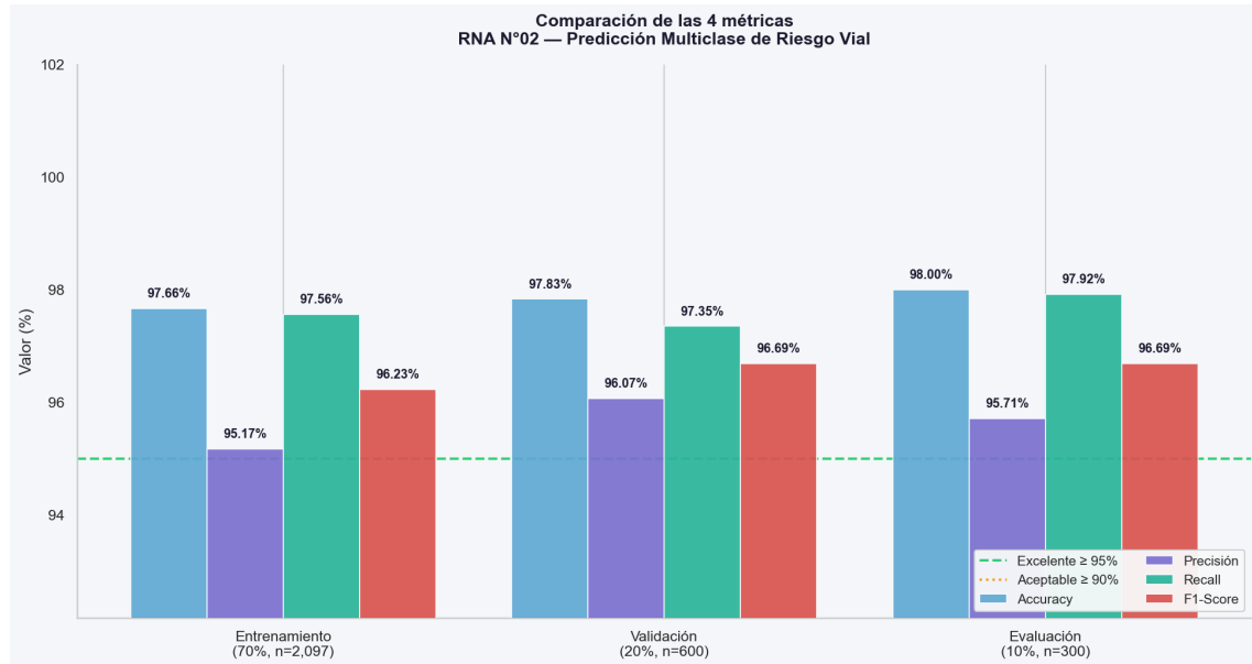
Figura 218 Comparación de las 4 métricas por partición — RNA N°02.
