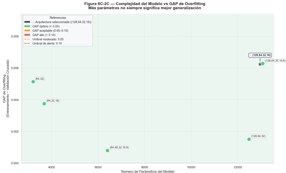
Figura 171 GAP vs número de parámetros de la RNA.
