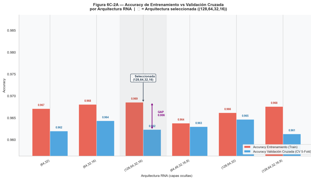
Figura 169 Accuracy vs por arquitectura RNA.
