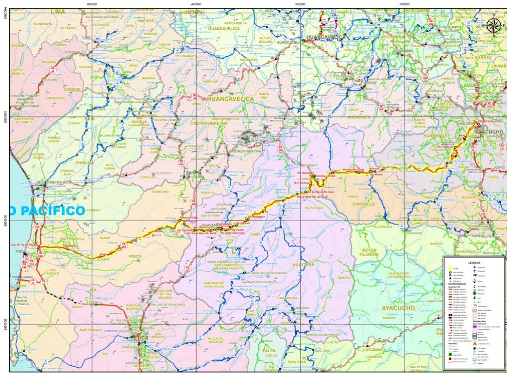
Figura 10 Plano de la Carretera Vía Los Libertadores (PE-28A)
