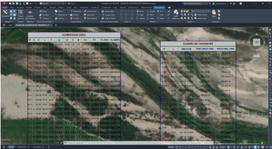
Figura 136 Modelamiento en el Civil 3D: Datos geometricos exportados. Fuente: Elaboración propia
