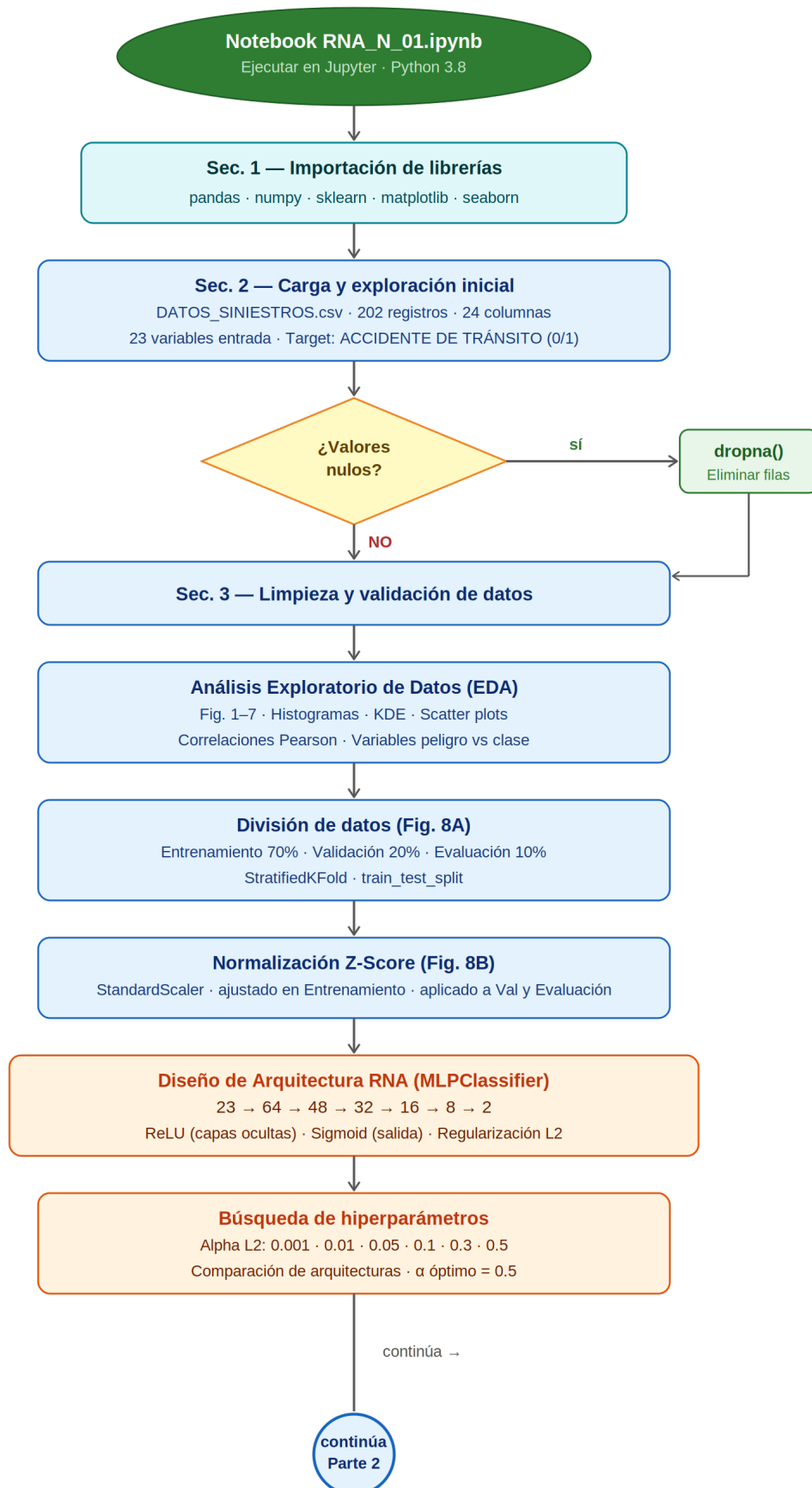
Figura 56 Diagrama de flujo de la RNA N°01 - Parte 1
