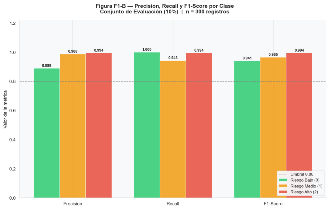
Figura 177 Precision, Recall y F1 por clase. Fuente: Elaboración propia
