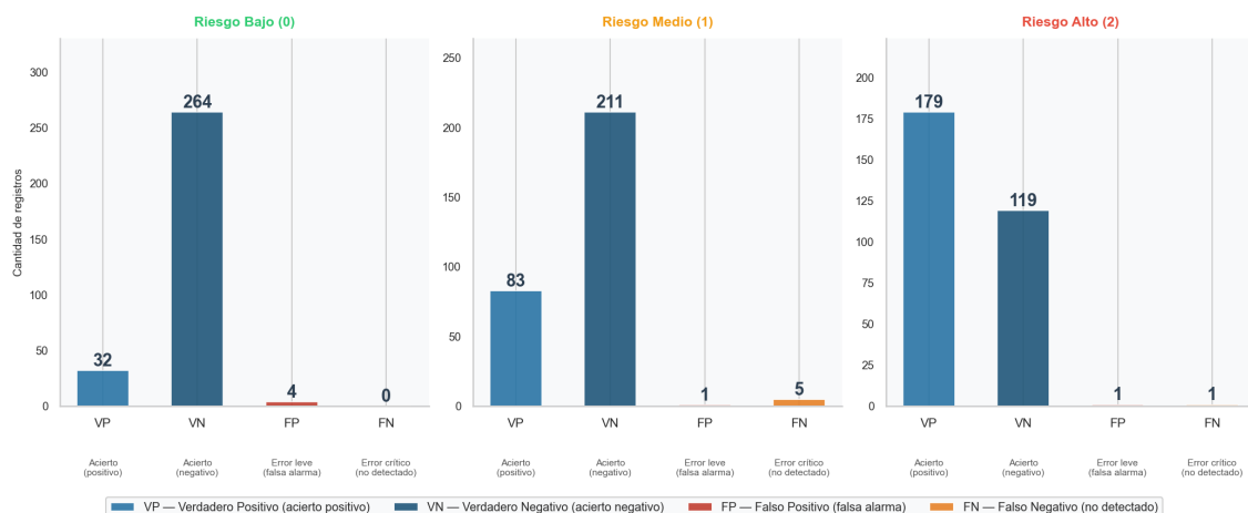
Figura 181 VP/VN/FP/FN por clase.
