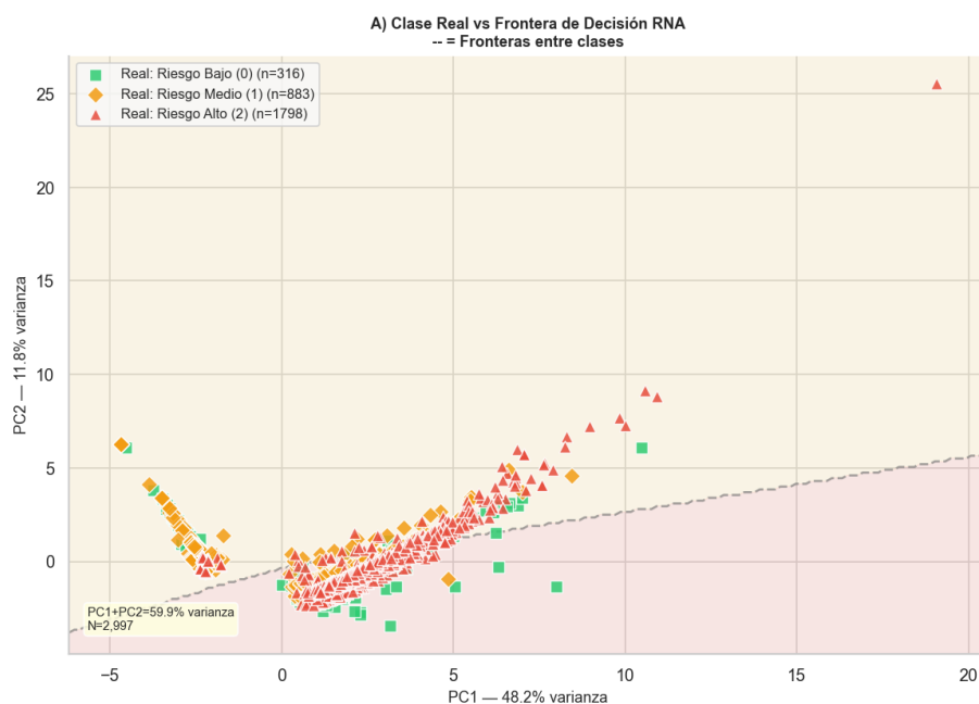
Figura 219 Clase real vs frontera de decisión del RNA.
