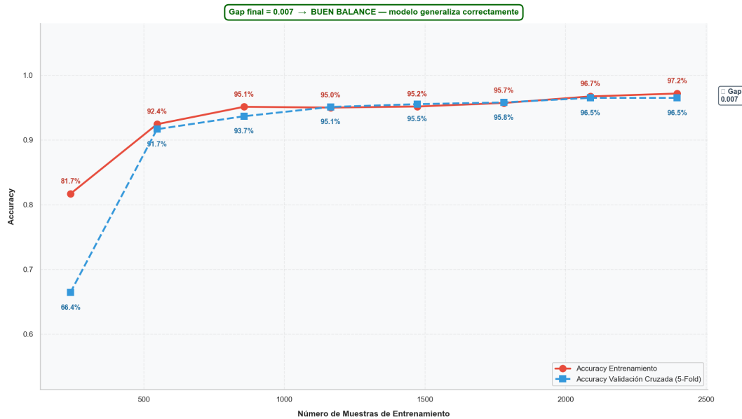
Figura 183 Curva de Aprendizaje: Diagnóstico de Bias Varianza del Modelo RNA
