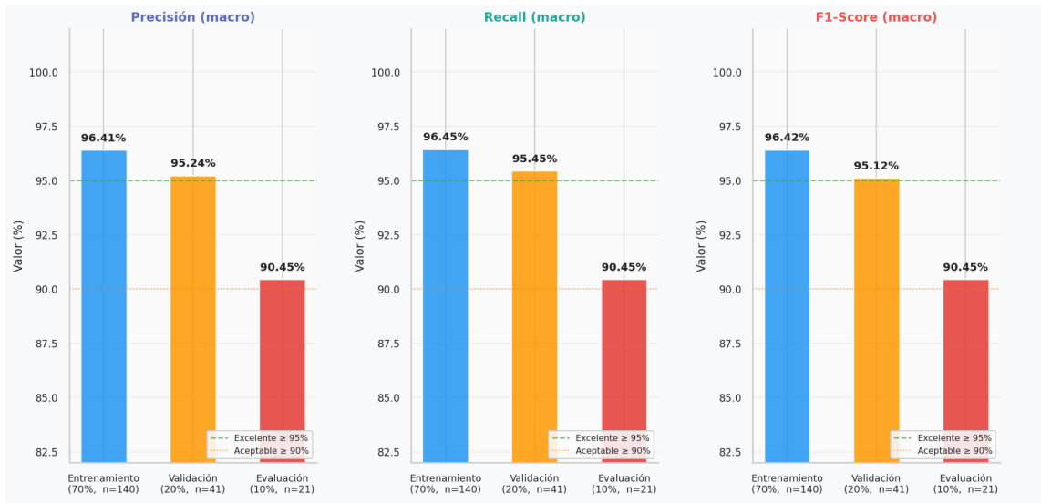
Figura 118 Precisión, Recall y F1-Score macro por partición. Fuente: Elaboración propia
