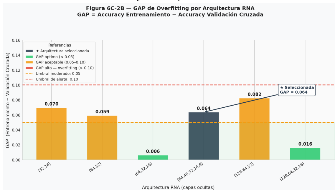
Figura 99 GAP de Overfitting por arquitectura.
