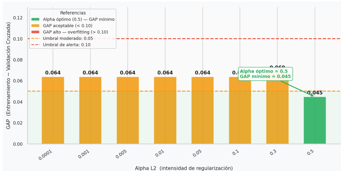
Figura 97 GAP de overfitting por valor de alpha.
