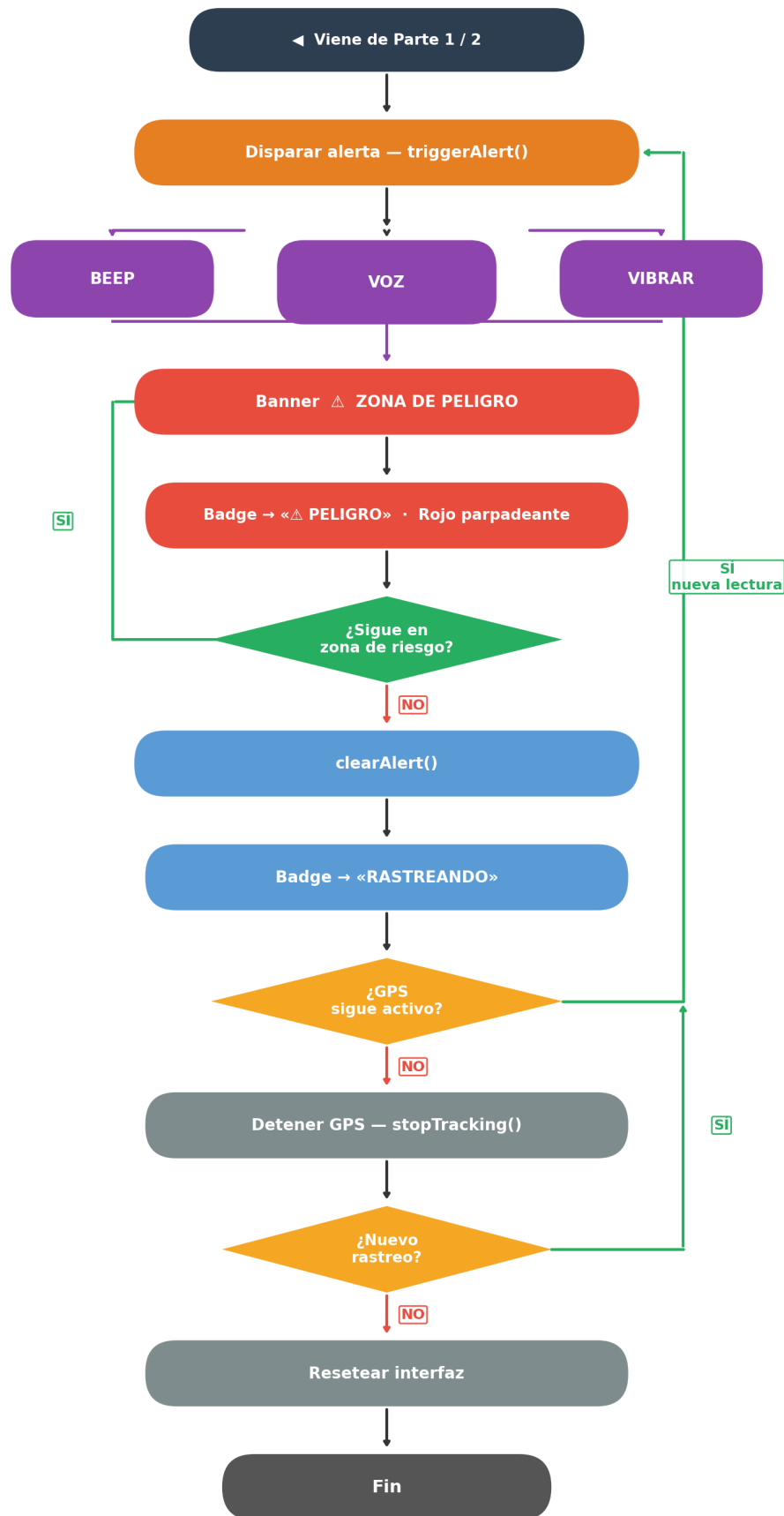
Figura 198 Diagrama de flujo - Parte II.
