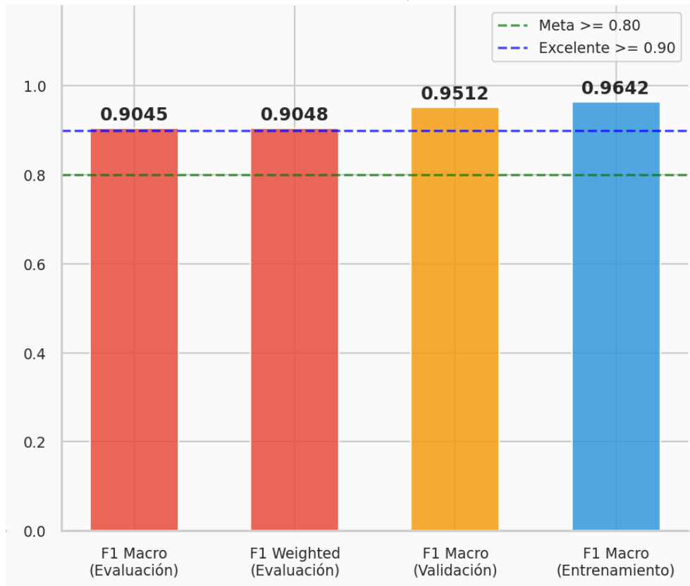
Figura 107 Resumen Global del F1-Score
