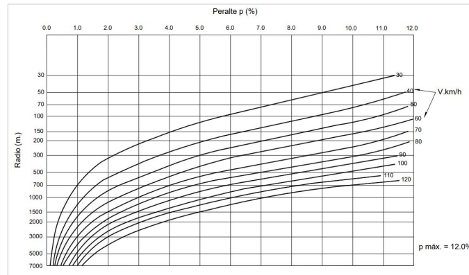
Figura 43 Peralte en zona rural (Tipo 3 ó 4)
