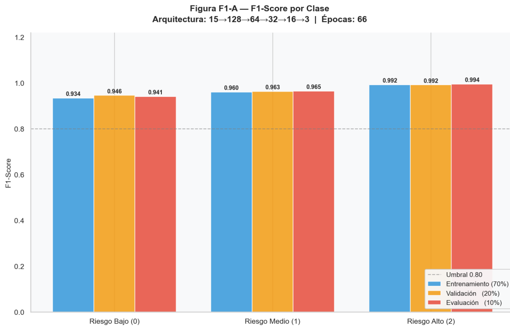
Figura 176 F1 Score por clase.
