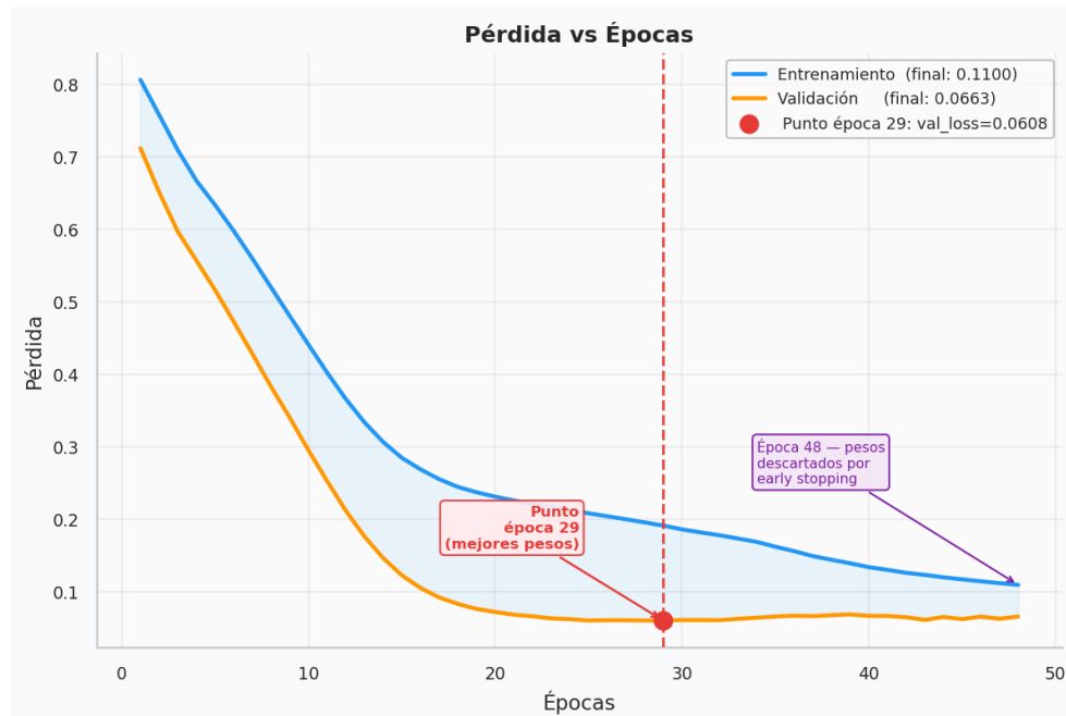
Figura 103 Pérdida (loss) vs. Épocas
