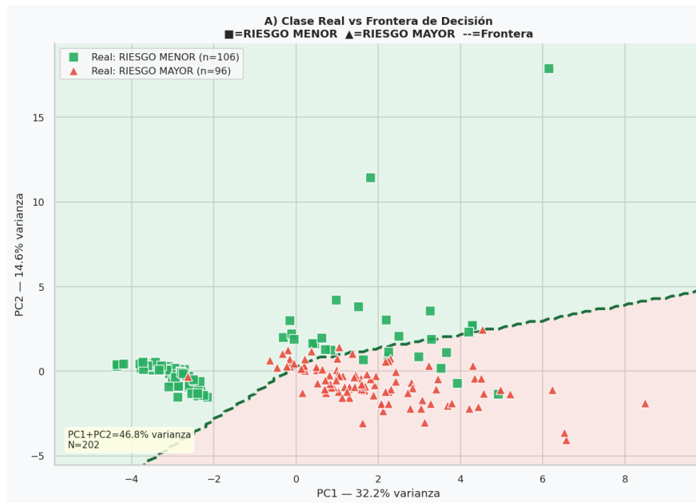
Figura 114 Clase Real vs Frontera de Decisión.
