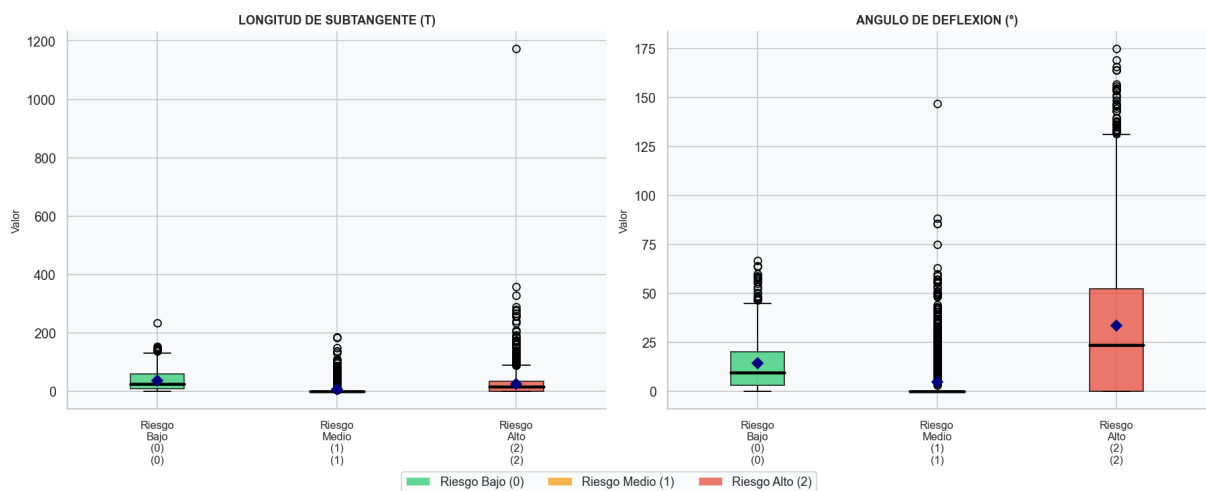
Figura 146 Boxplots de variables de Longitud de subtangente y angulo de deflexión.
