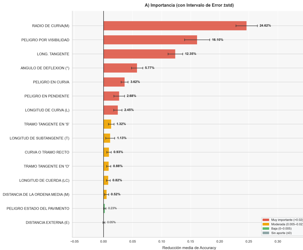
Figura 184 Importancia de variables con intervalo de error.
