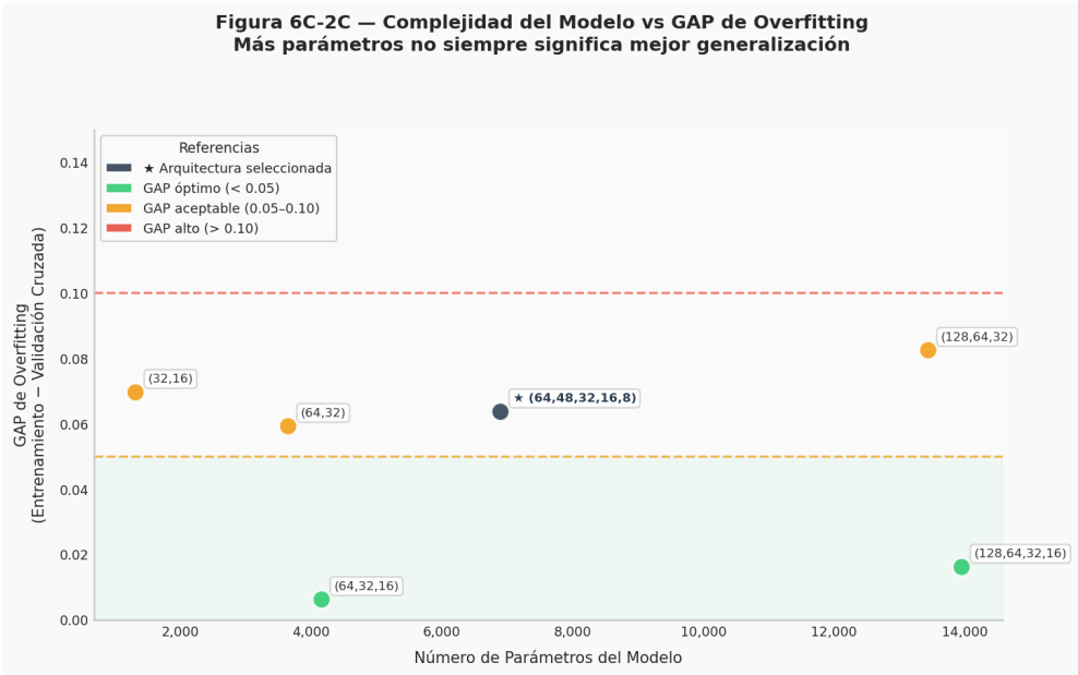
Figura 100 GAP de Overfitting vs Número de parámetros de la arquitectura. Fuente: Elaboración propia
