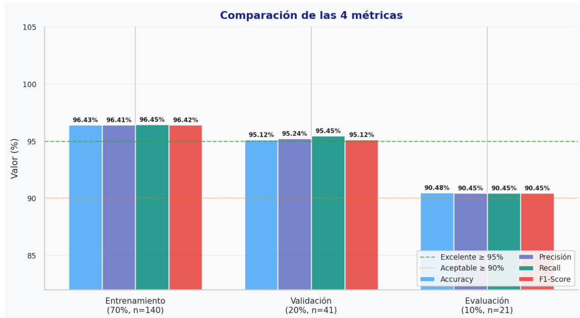
Figura 119 Comparación de las 4 métricas por partición.
