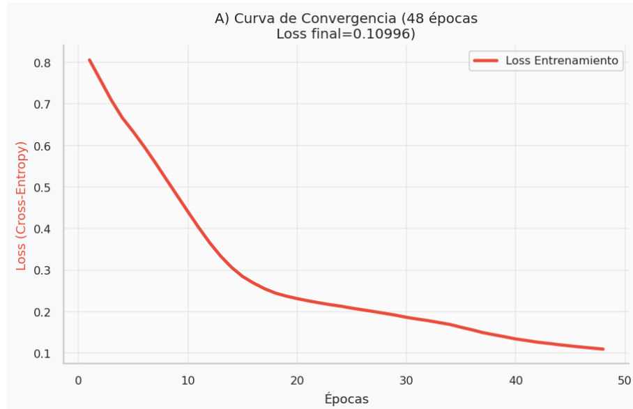
Figura 101 Curva de convergencia: Perdida vs Epocas.
