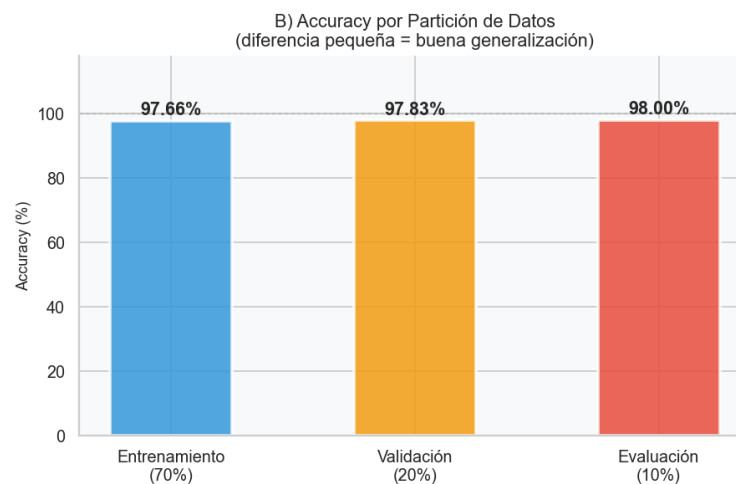
Figura 173 Accuracy por partición.
