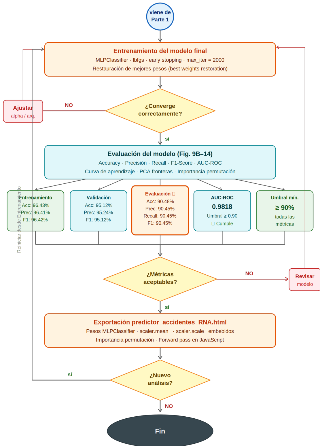
Figura 57 Diagrama de flujo de la RNA N°01 - Parte 2
