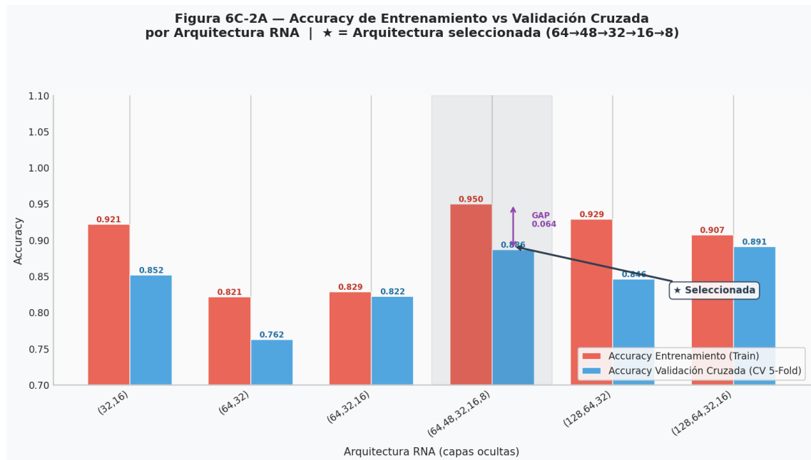
Figura 98 Accuracy de entrenamiento y validación cruzada por arquitectura.
